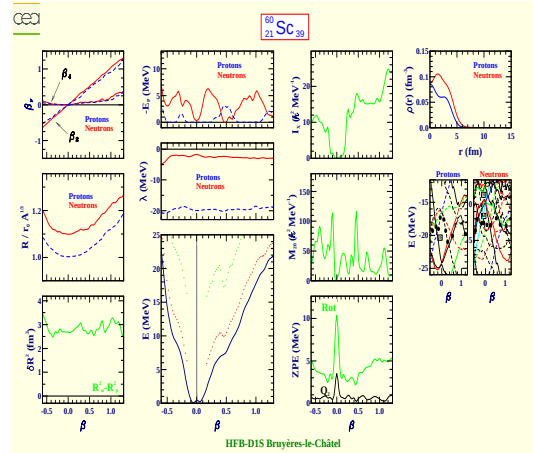
Scandium 60 (Z=21, N=39)
