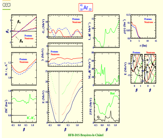
Argon 41 (Z=18, N=23)
