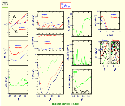
Argon 53 (Z=18, N=35)
