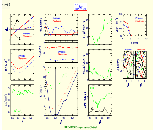
Argon 47 (Z=18, N=29)
