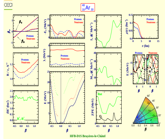
Argon 48 (Z=18, N=30)
