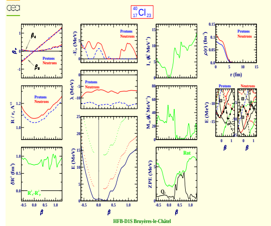
Chlorine 40 (Z=17, N=23)
