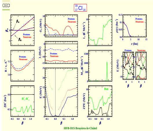
Chlorine 33 (Z=17, N=16)
