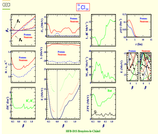
Chlorine 51 (Z=17, N=34)
