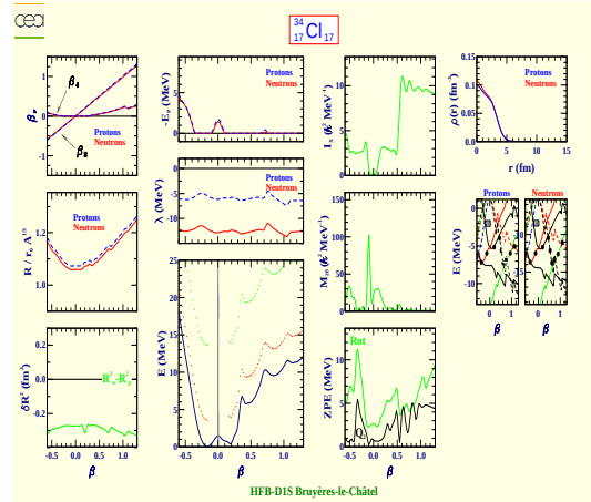
Chlorine 34 (Z=17, N=17)
