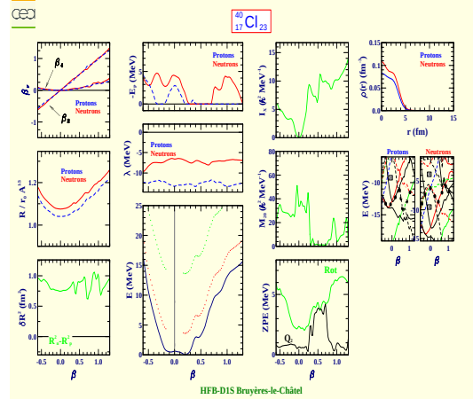
Chlore 40 (Z=17, N=23)
