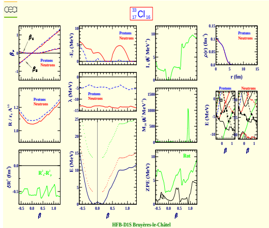
Chlore 33 (Z=17, N=16)
