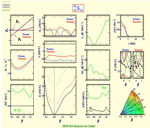
Soufre 36 (Z=16, N=20)
