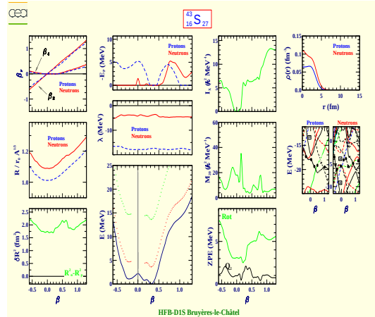
Soufre 43 (Z=16, N=27)
