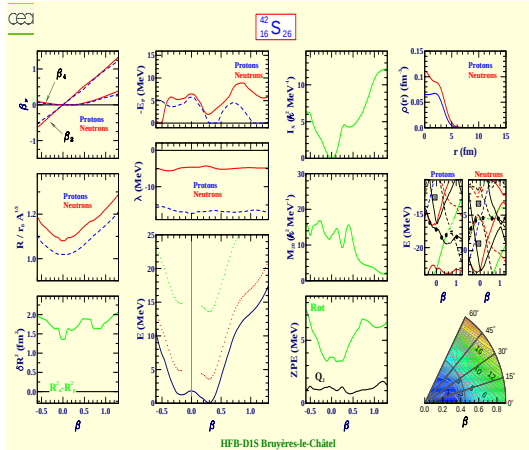
Soufre 42 (Z=16, N=26)
