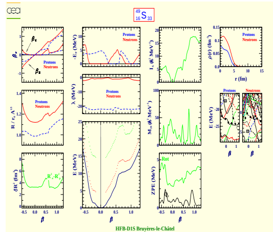
Soufre 49 (Z=16, N=33)
