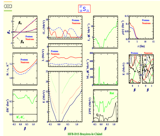
Soufre 37 (Z=16, N=21)
