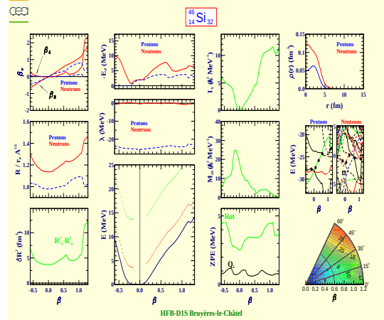
Silicon 46 (Z=14, N=32)
