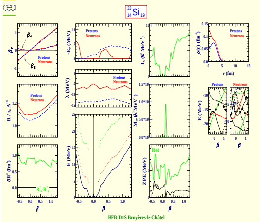
Silicon 33 (Z=14, N=19)
