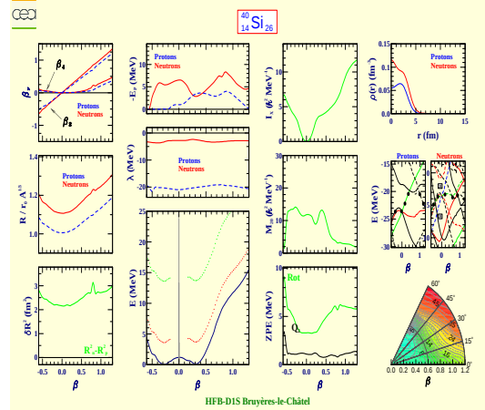
Silicon 40 (Z=14, N=26)
