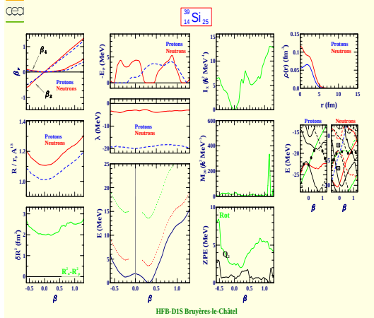
Silicon 39 (Z=14, N=25)
