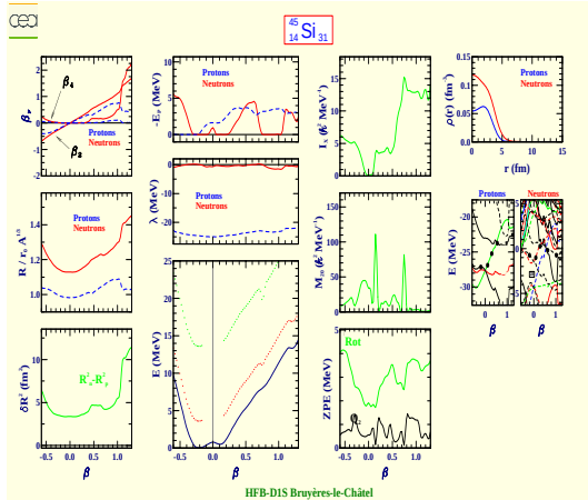
Silicium 45 (Z=14, N=31)
