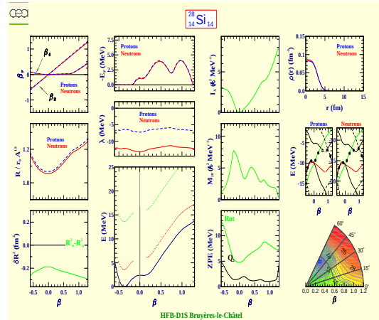
Silicium 28 (Z=14, N=14)
