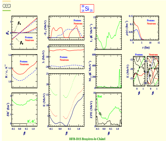
Silicium 39 (Z=14, N=25)
