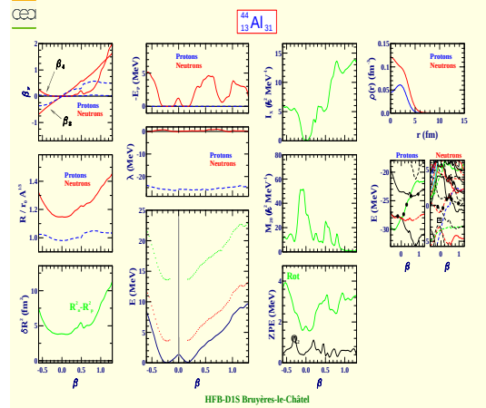
Aluminium 44 (Z=13, N=31)
