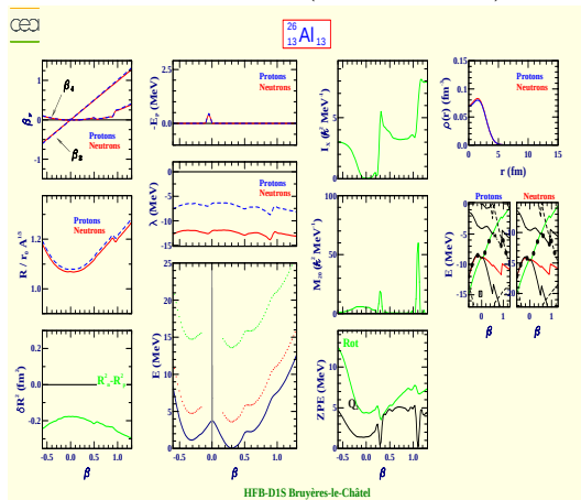
Aluminium 26 (Z=13, N=13)
