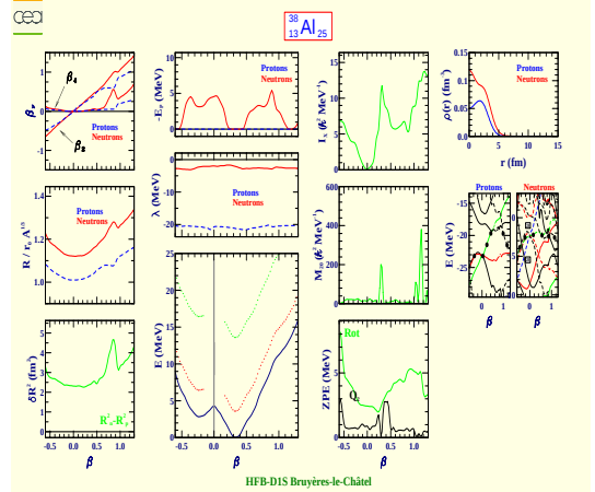
Aluminium 38 (Z=13, N=25)
