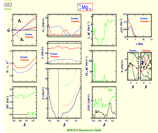
Magnesium 31 (Z=12, N=19)
