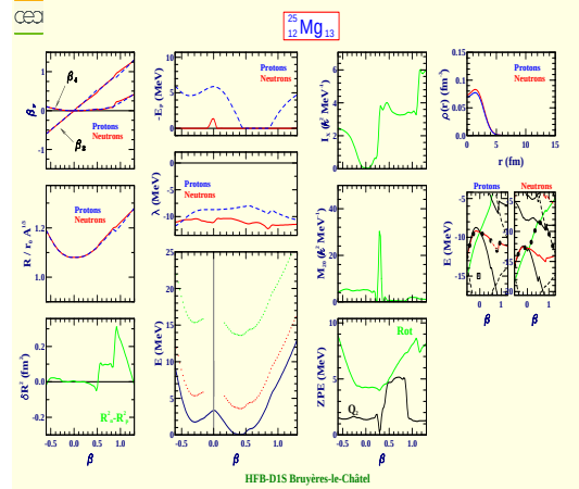
Magnesium 25 (Z=12, N=13)
