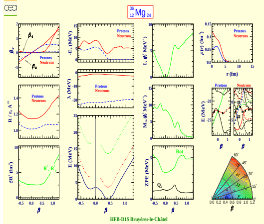
Magnésium 36 (Z=12, N=24)
