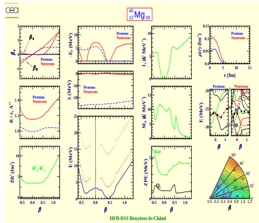
Magnésium 40 (Z=12, N=28)
