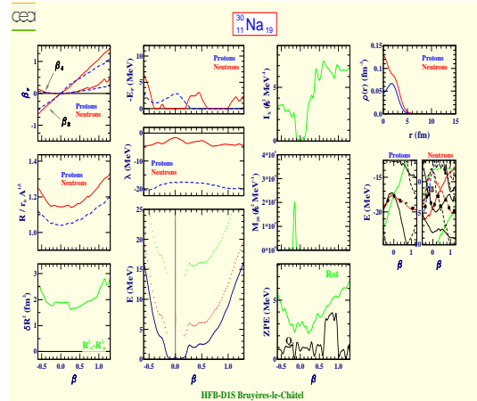
Sodium 30 (Z=11, N=19)
