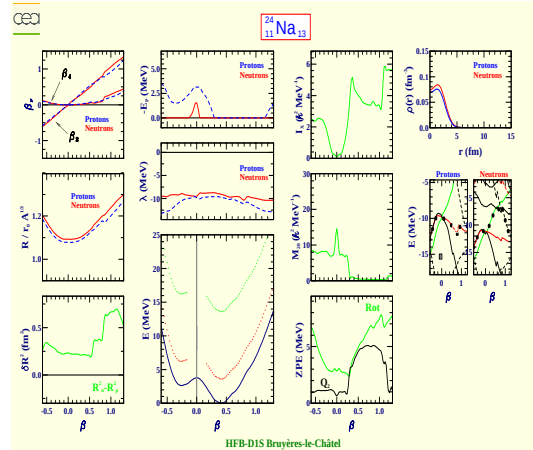
Sodium 24 (Z=11, N=13)
