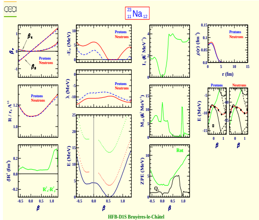
Sodium 23 (Z=11, N=12)
