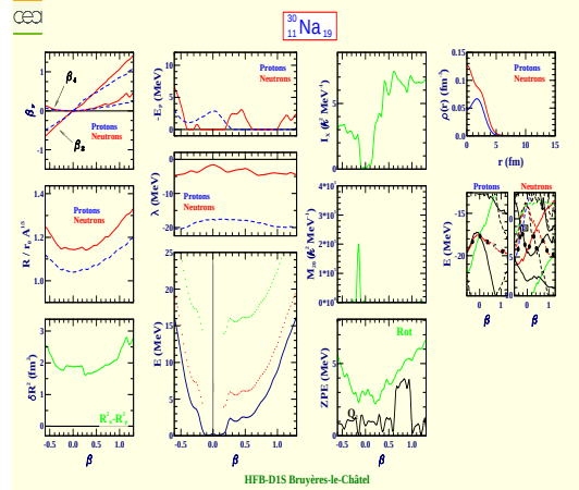
Sodium 30 (Z=11, N=19)
