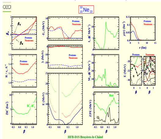
Neon 33 (Z=10, N=23)
