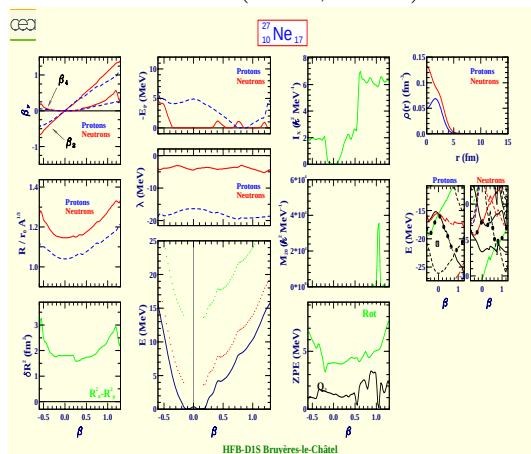
Neon 27 (Z=10, N=17)
