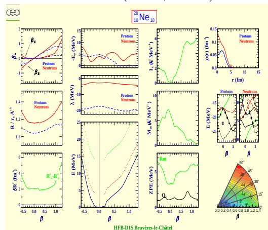
Neon 28 (Z=10, N=18)
