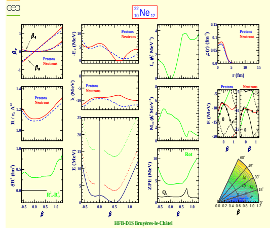
Néon 22 (Z=10, N=12)
