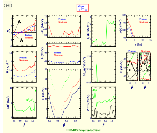
Fluor 26 (Z=9, N=17)
