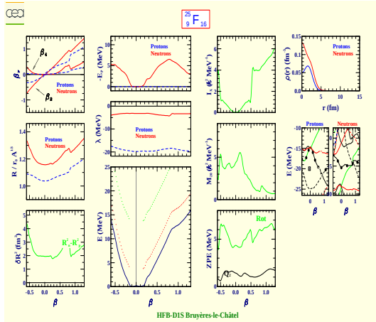
Fluor 25 (Z=9, N=16)
