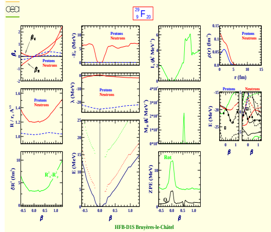
Fluor 29 (Z=9, N=20)
