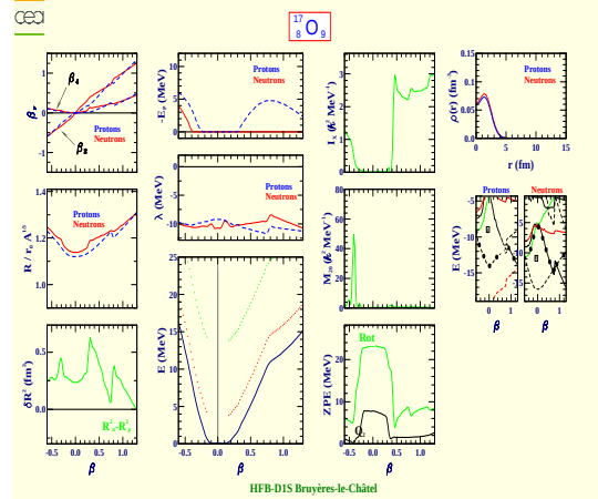
Oxygen 17 (Z=8, N=9)
