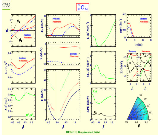
Oxygène 22 (Z=8, N=14)
