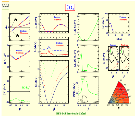
Oxygène 16 (Z=8, N=8)
