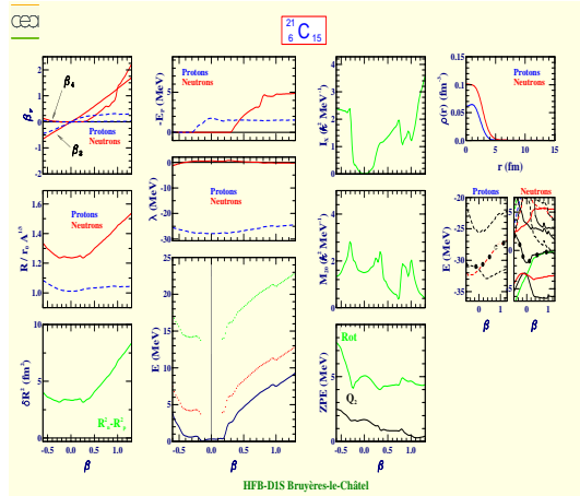
Carbone 21 (Z=6, N=15)
