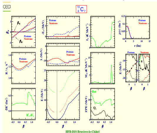
Carbone 13 (Z=6, N=7)
