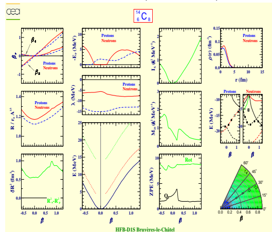
Carbone 14 (Z=6, N=8)
