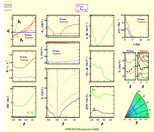
Carbone 22 (Z=6, N=16)
