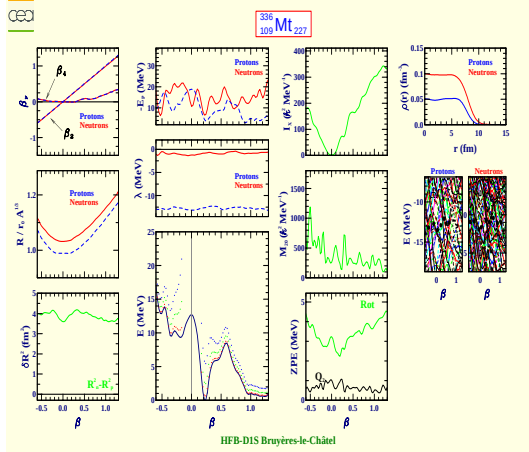
Meitnerium 336 (Z=109, N=227)
