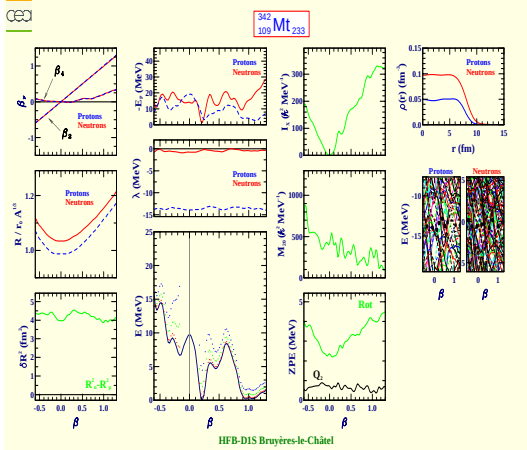
Meitnerium 342 (Z=109, N=233)
