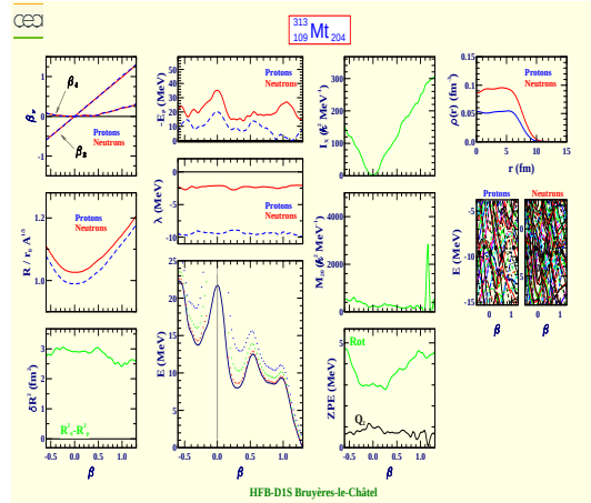
Meitnerium 313 (Z=109, N=204)
