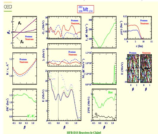
Meitnerium 283 (Z=109, N=174)
