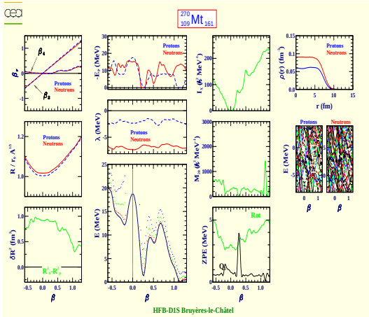
Meitnerium 270 (Z=109, N=161)
