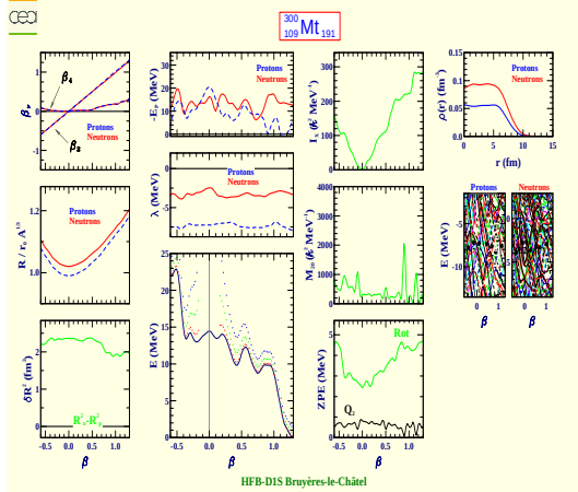
Meitnerium 300 (Z=109, N=191)
