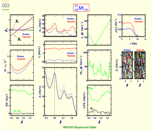
Meitnerium 312 (Z=109, N=203)
