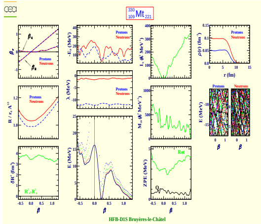
Meitnerium 330 (Z=109, N=221)
