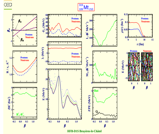
Meitnerium 319 (Z=109, N=210)
