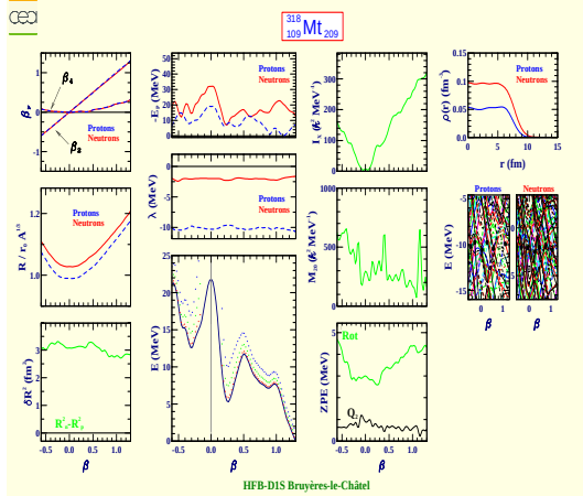
Meitnerium 318 (Z=109, N=209)
