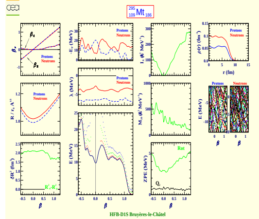
Meitnerium 295 (Z=109, N=186)
