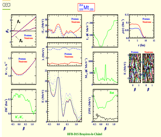
Meitnerium 264 (Z=109, N=155)
