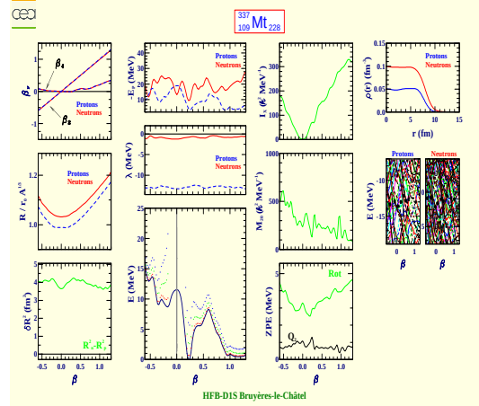
Meitnerium 337 (Z=109, N=228)
