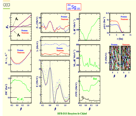
Seaborgium 261 (Z=106, N=155)
