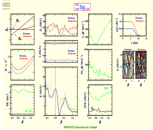
Seaborgium 332 (Z=106, N=226)
