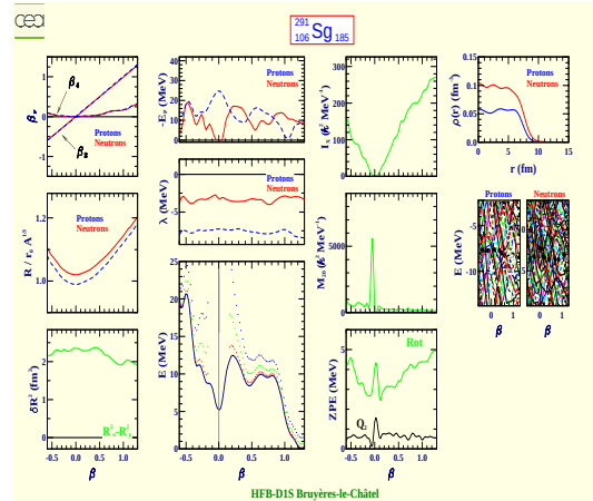
Seaborgium 291 (Z=106, N=185)
