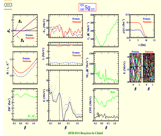
Seaborgium 333 (Z=106, N=227)
