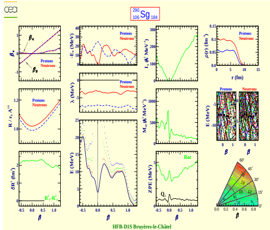
Seaborgium 290 (Z=106, N=184)
