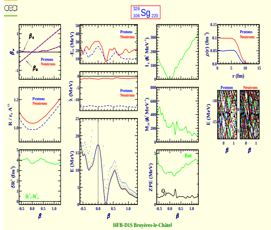
Seaborgium 326 (Z=106, N=220)
