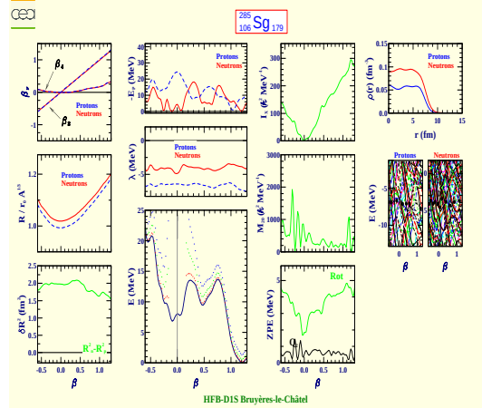
Seaborgium 285 (Z=106, N=179)
