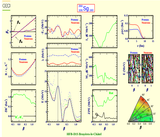
Seaborgium 266 (Z=106, N=160)
