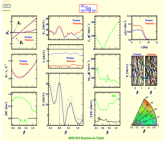
Seaborgium 260 (Z=106, N=154)
