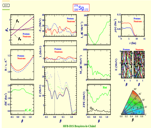
Seaborgium 278 (Z=106, N=172)
