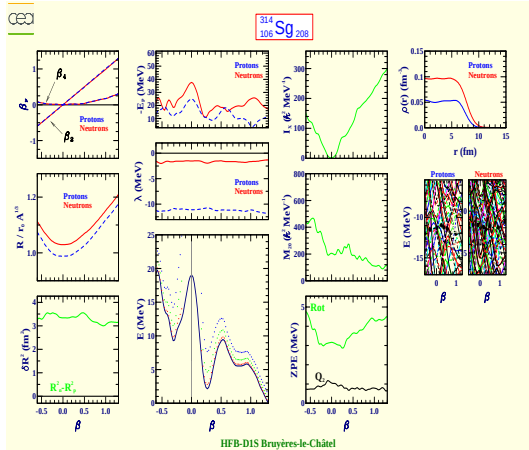
Seaborgium 314 (Z=106, N=208)
