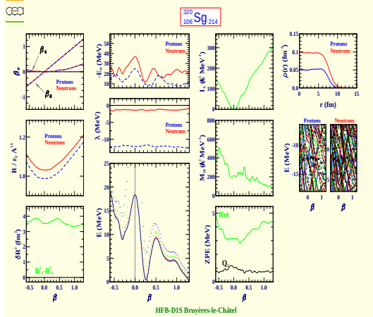
Seaborgium 320 (Z=106, N=214)
