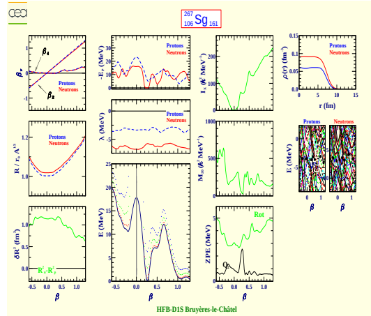
Seaborgium 267 (Z=106, N=161)
