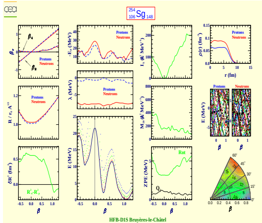
Seaborgium 254 (Z=106, N=148)
