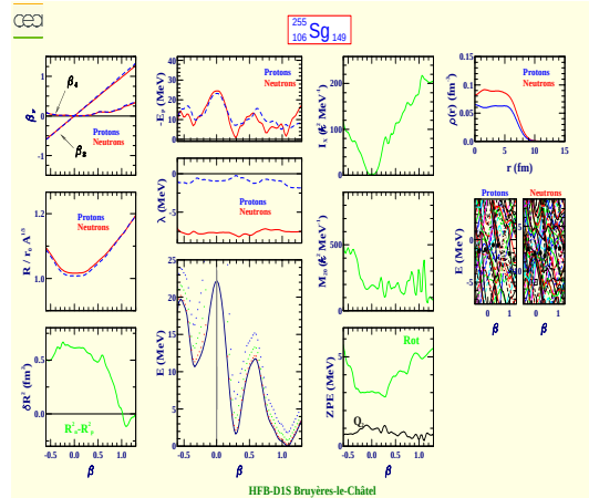
Seaborgium 255 (Z=106, N=149)
