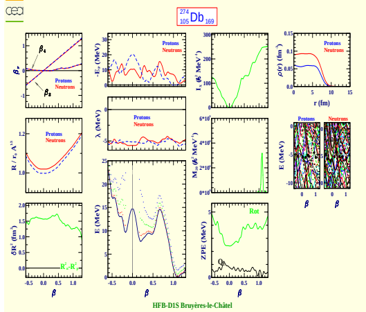
Dubnium 274 (Z=105, N=169)
