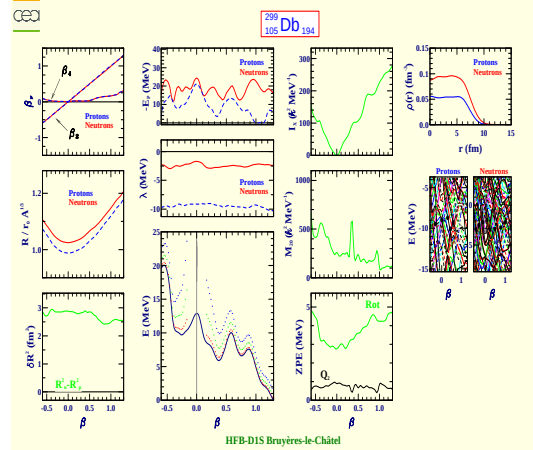
Dubnium 299 (Z=105, N=194)
