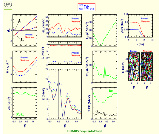
Dubnium 323 (Z=105, N=218)
