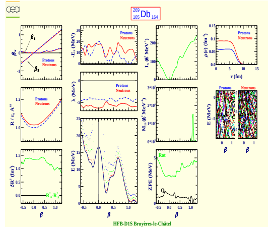
Dubnium 269 (Z=105, N=164)
