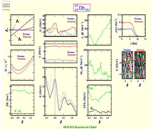
Dubnium 310 (Z=105, N=205)
