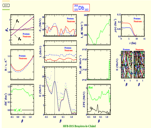
Dubnium 268 (Z=105, N=163)
