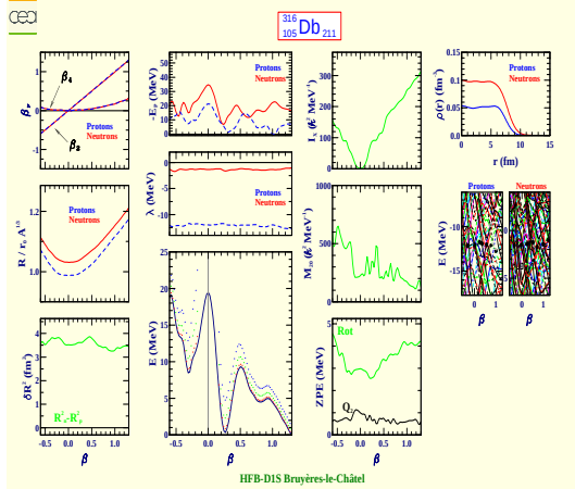
Dubnium 316 (Z=105, N=211)
