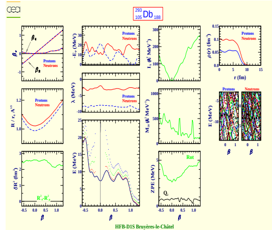
Dubnium 293 (Z=105, N=188)
