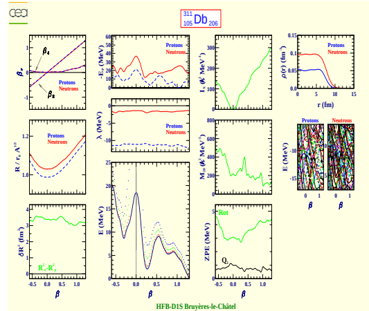
Dubnium 311 (Z=105, N=206)
