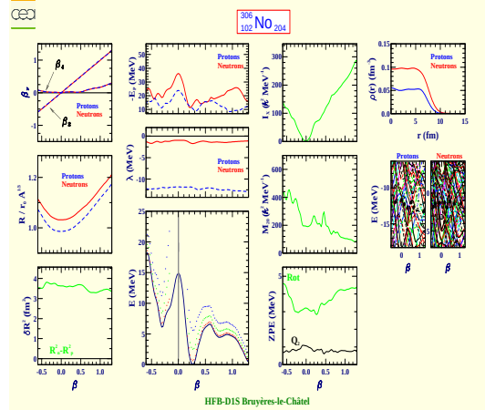
Nobelium 306 (Z=102, N=204)
