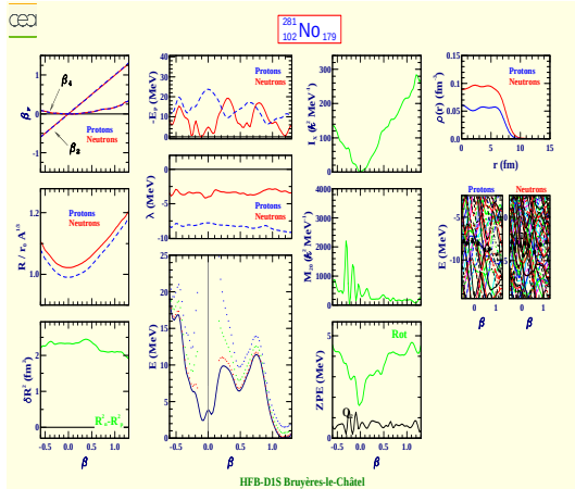
Nobelium 281 (Z=102, N=179)
