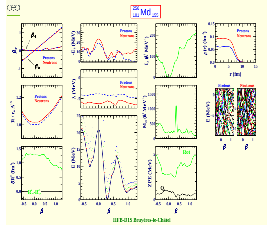
Mendelevium 256 (Z=101, N=155)
