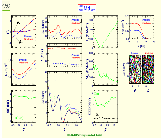
Mendelevium 303 (Z=101, N=202)
