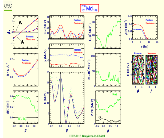
Mendelevium 250 (Z=101, N=149)
