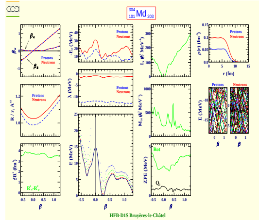
Mendelevium 304 (Z=101, N=203)
