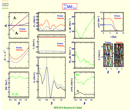
Mendelevium 315 (Z=101, N=214)
