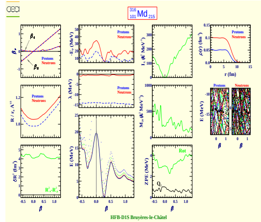
Mendelevium 316 (Z=101, N=215)
