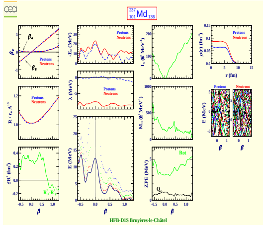
Mendelevium 237 (Z=101, N=136)
