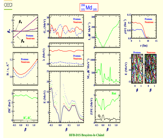
Mendelevium 286 (Z=101, N=185)
