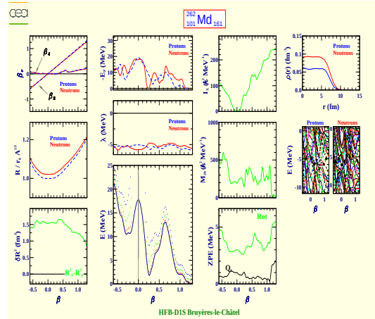
Mendelevium 262 (Z=101, N=161)
