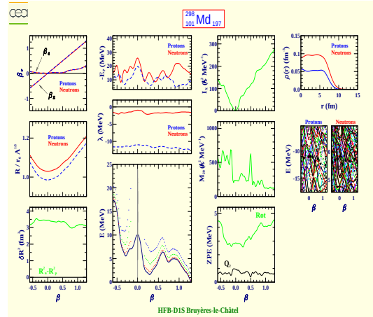
Mendelevium 298 (Z=101, N=197)
