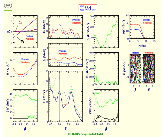
Mendelevium 268 (Z=101, N=167)
