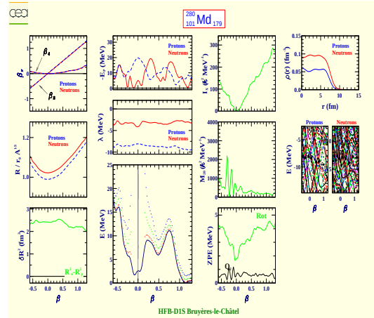
Mendelevium 280 (Z=101, N=179)
