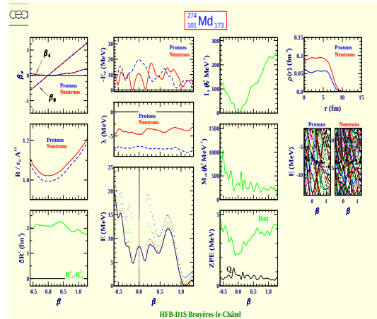
Mendelevium 274 (Z=101, N=173)
