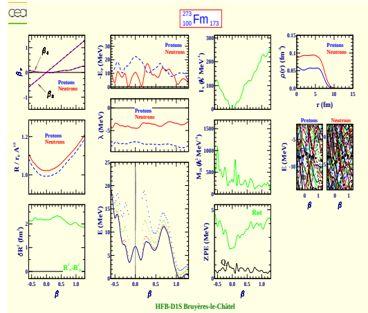
Fermium 273 (Z=100, N=173)
