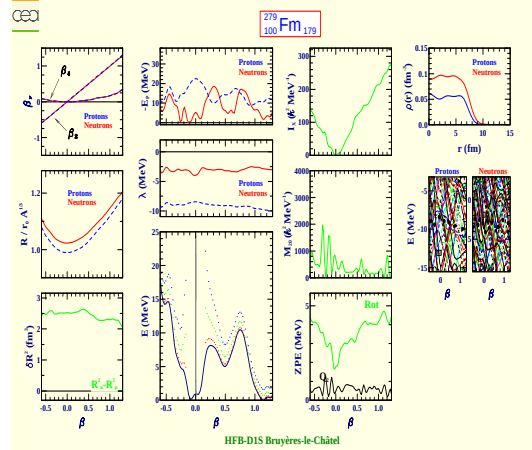
Fermium 279 (Z=100, N=179)
