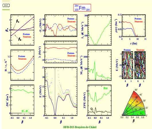
Fermium 284 (Z=100, N=184)
