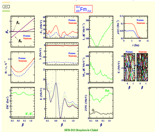
Fermium 314 (Z=100, N=214)
