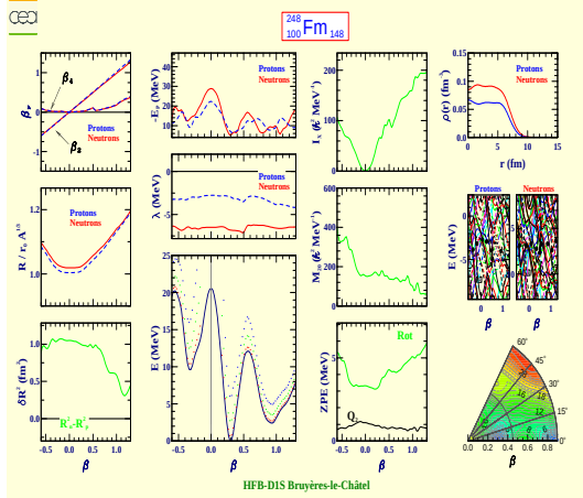
Fermium 248 (Z=100, N=148)
