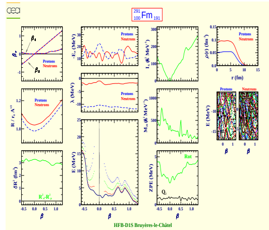
Fermium 291 (Z=100, N=191)
