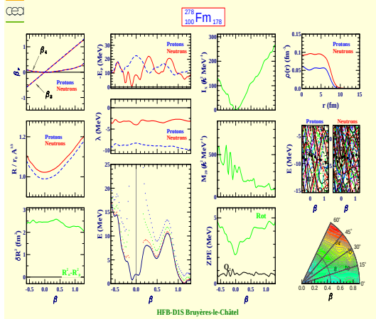
Fermium 278 (Z=100, N=178)
