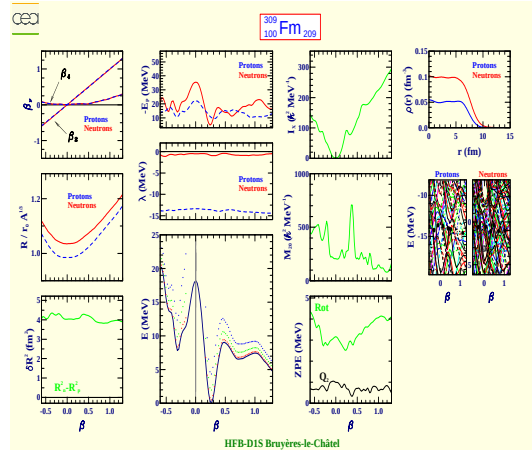
Fermium 309 (Z=100, N=209)
