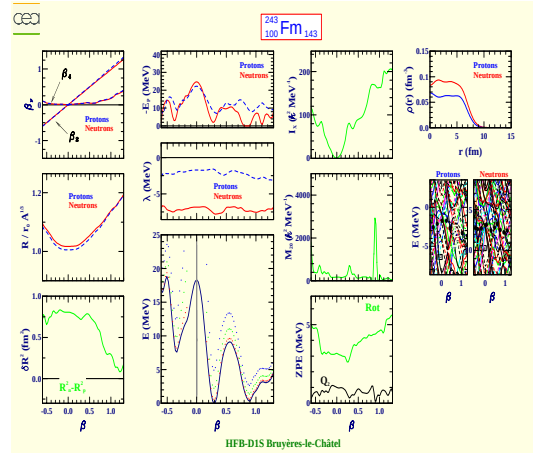
Fermium 243 (Z=100, N=143)
