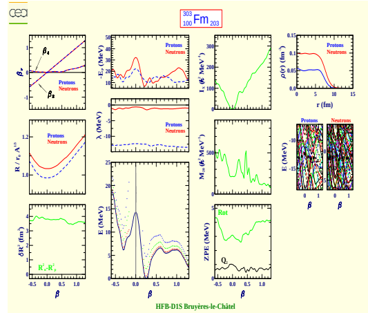
Fermium 303 (Z=100, N=203)
