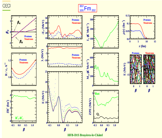
Fermium 302 (Z=100, N=202)
