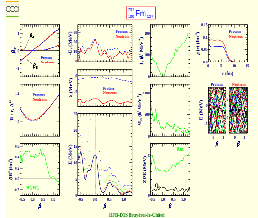
Fermium 237 (Z=100, N=137)
