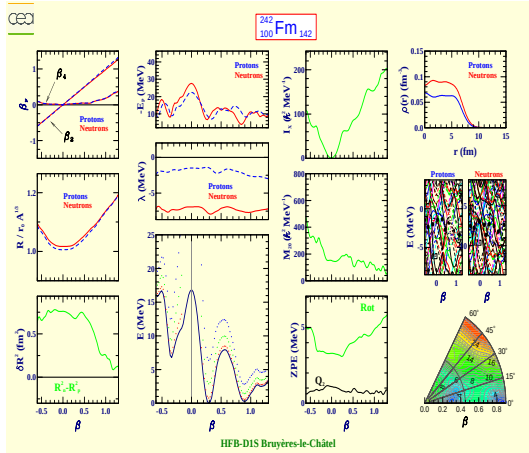
Fermium 242 (Z=100, N=142)
