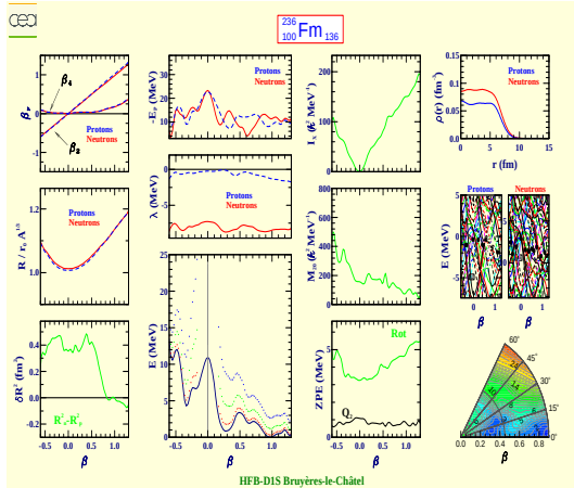
Fermium 236 (Z=100, N=136)
