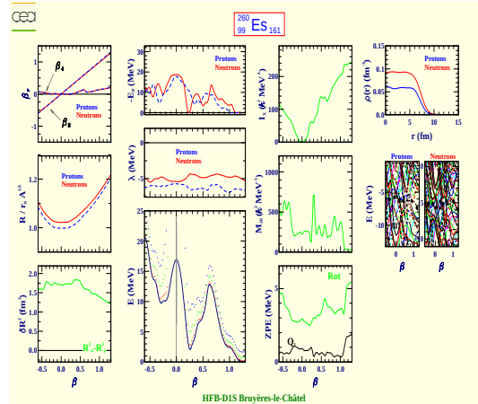
Einsteinium 260 (Z=99, N=161)
