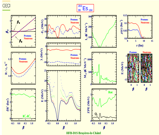
Einsteinium 283 (Z=99, N=184)
