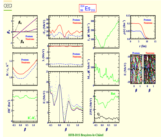
Einsteinium 314 (Z=99, N=215)
