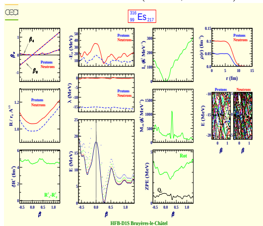
Einsteinium 316 (Z=99, N=217)
