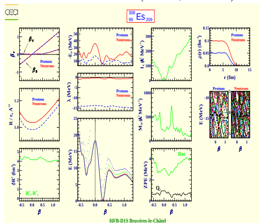
Einsteinium 308 (Z=99, N=209)
