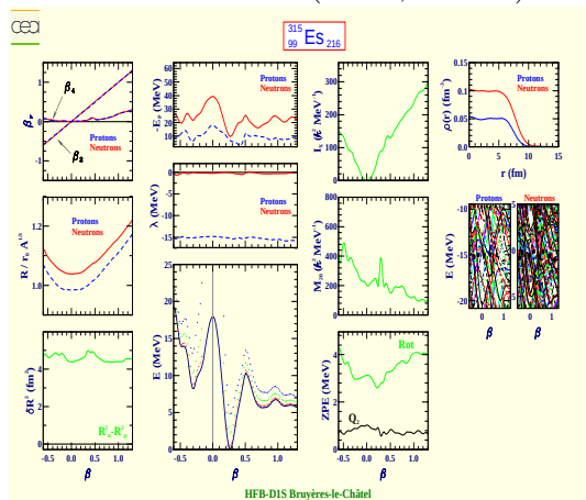
Einsteinium 315 (Z=99, N=216)
