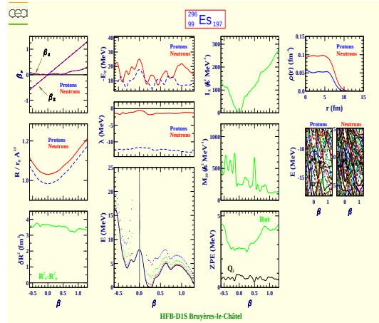
Einsteinium 296 (Z=99, N=197)
