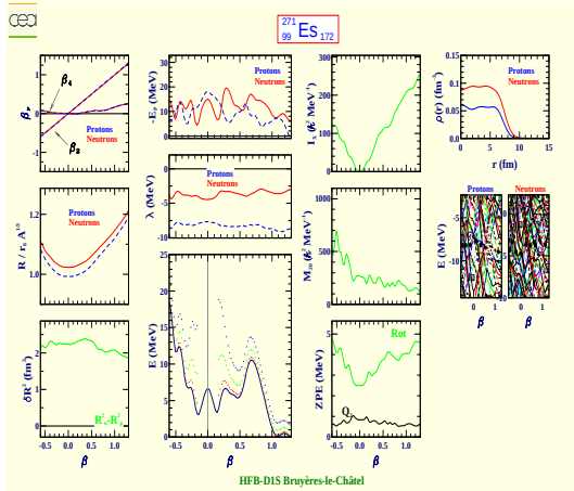
Einsteinium 271 (Z=99, N=172)
