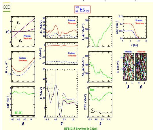
Einsteinium 307 (Z=99, N=208)
