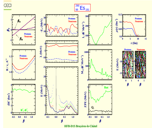
Einsteinium 290 (Z=99, N=191)
