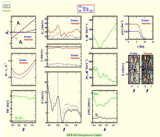
Einsteinium 301 (Z=99, N=202)
