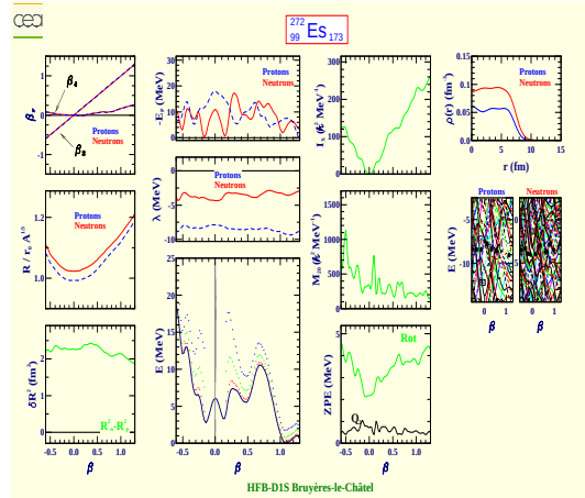
Einsteinium 272 (Z=99, N=173)
