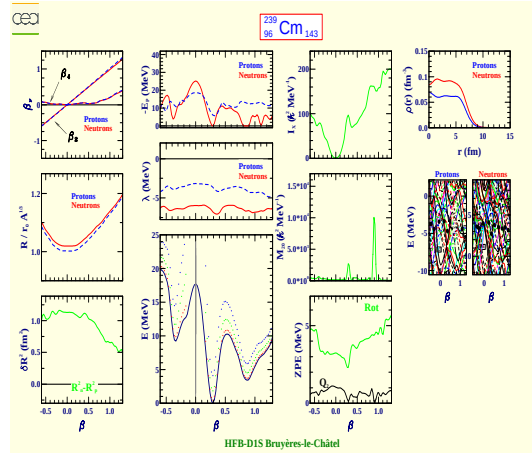
Curium 239 (Z=96, N=143)
