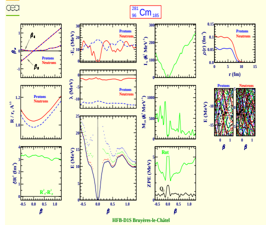
Curium 281 (Z=96, N=185)
