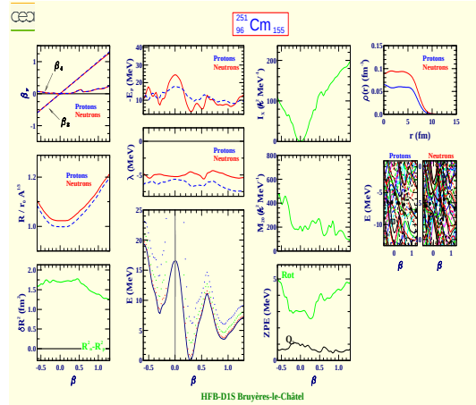
Curium 251 (Z=96, N=155)
