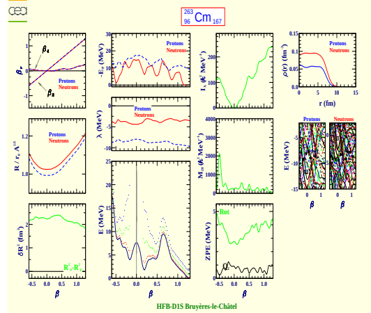
Curium 263 (Z=96, N=167)
