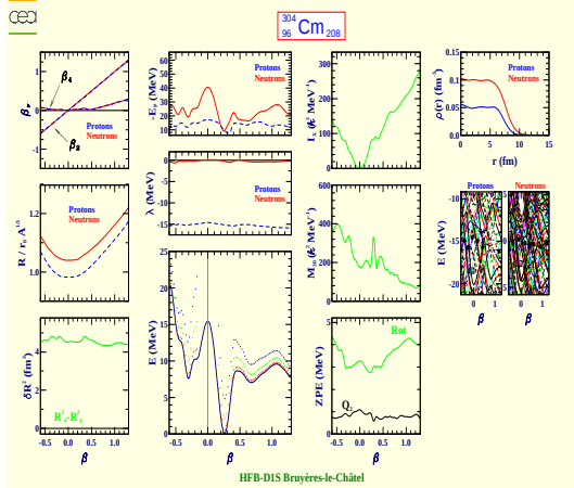
Curium 304 (Z=96, N=208)
