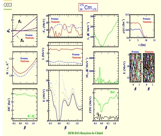
Curium 275 (Z=96, N=179)
