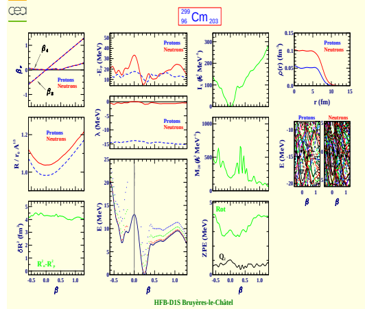
Curium 299 (Z=96, N=203)
