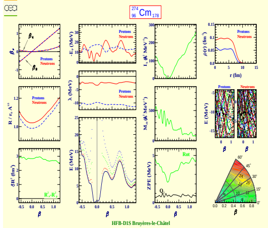
Curium 274 (Z=96, N=178)
