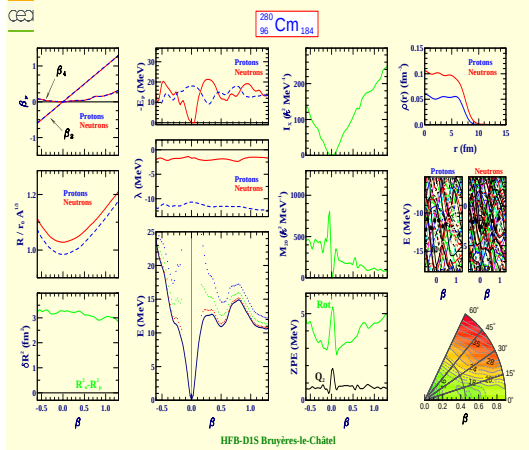
Curium 280 (Z=96, N=184)
