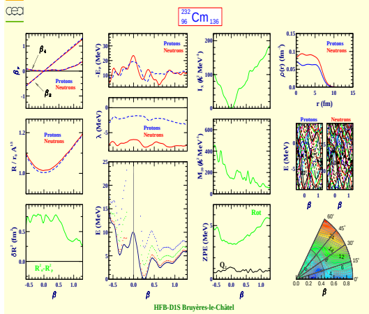
Curium 232 (Z=96, N=136)
