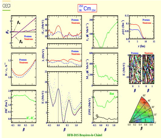
Curium 250 (Z=96, N=154)
