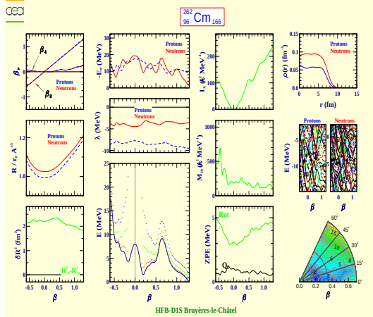
Curium 262 (Z=96, N=166)
