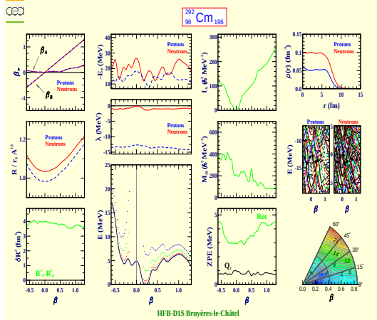
Curium 292 (Z=96, N=196)
