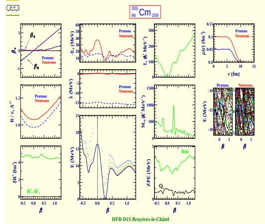
Curium 305 (Z=96, N=209)
