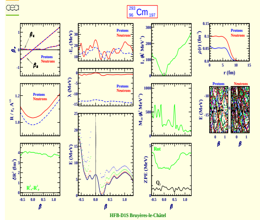
Curium 293 (Z=96, N=197)
