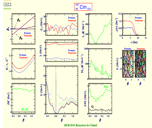
Curium 287 (Z=96, N=191)
