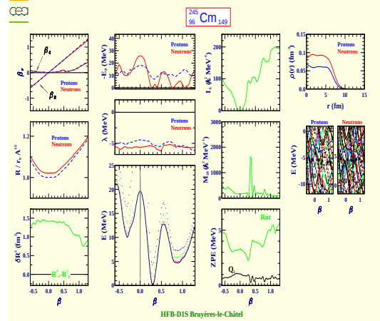
Curium 245 (Z=96, N=149)
