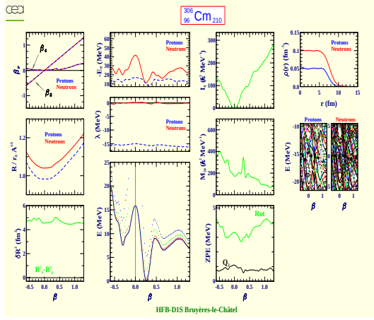
Curium 306 (Z=96, N=210)
