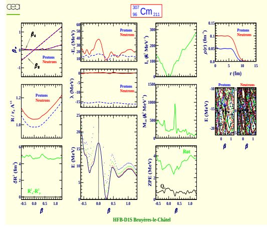
Curium 307 (Z=96, N=211)
