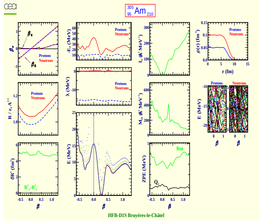
Americium 305 (Z=95, N=210)
