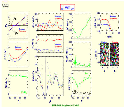
Americium 272 (Z=95, N=177)
