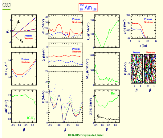
Americium 253 (Z=95, N=158)
