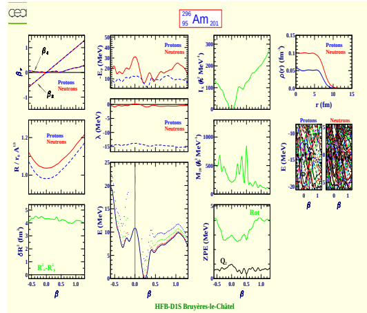
Americium 296 (Z=95, N=201)
