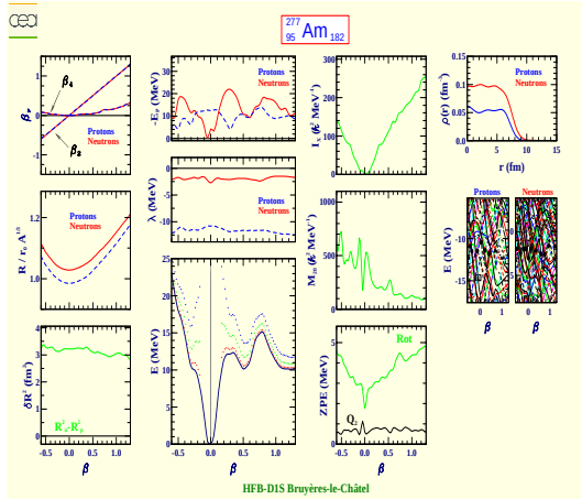
Americium 277 (Z=95, N=182)
