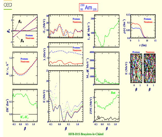
Americium 230 (Z=95, N=135)
