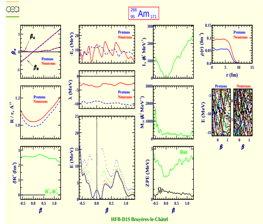
Americium 266 (Z=95, N=171)
