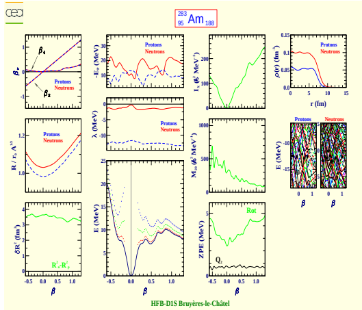
Americium 283 (Z=95, N=188)
