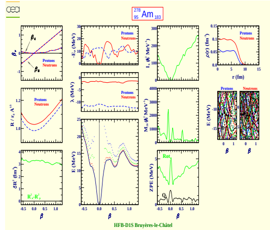
Americium 278 (Z=95, N=183)
