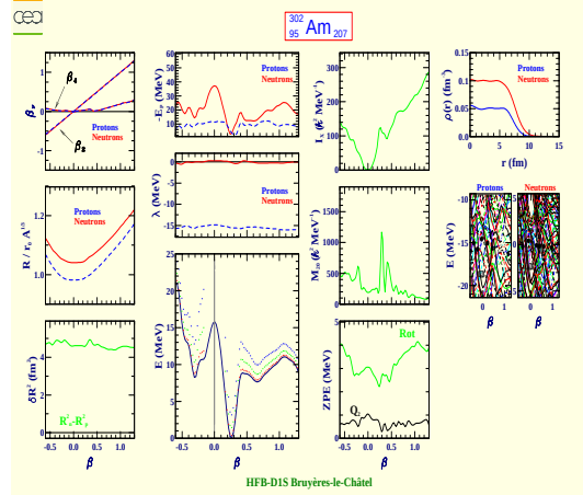
Americium 302 (Z=95, N=207)
