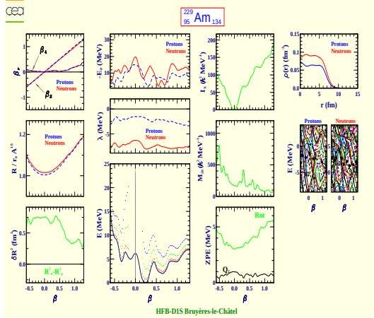
Americium 229 (Z=95, N=134)
