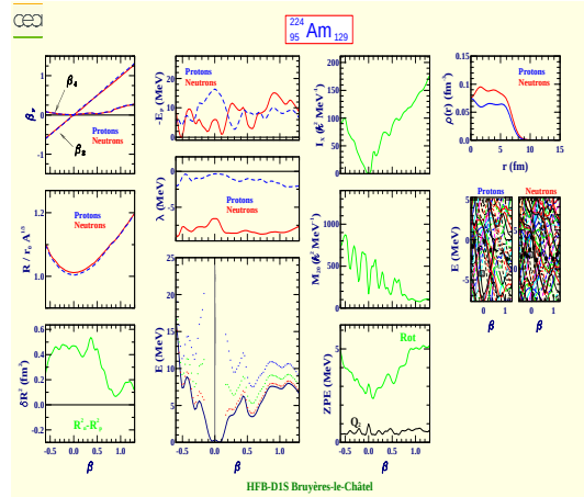
Americium 224 (Z=95, N=129)
