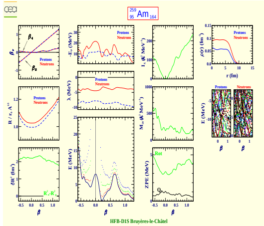
Americium 259 (Z=95, N=164)
