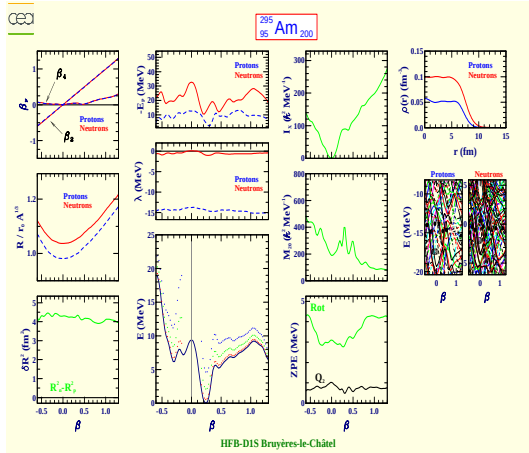
Americium 295 (Z=95, N=200)
