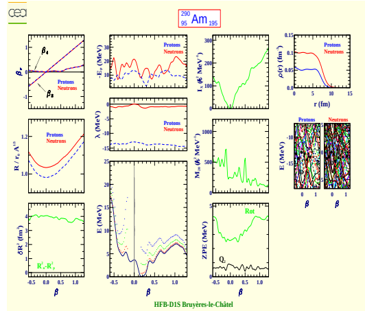
Americium 290 (Z=95, N=195)
