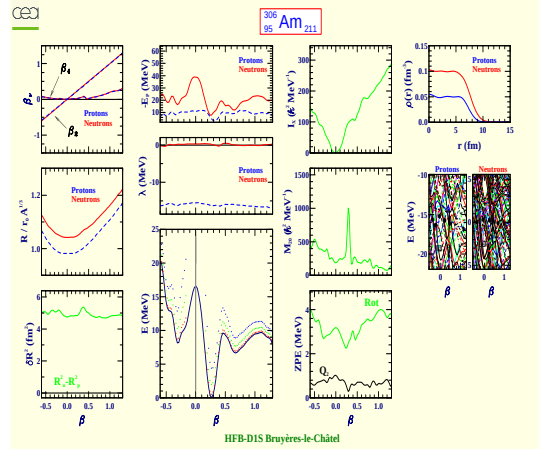
Americium 306 (Z=95, N=211)
