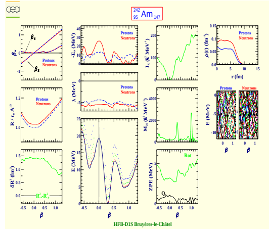
Americium 242 (Z=95, N=147)
