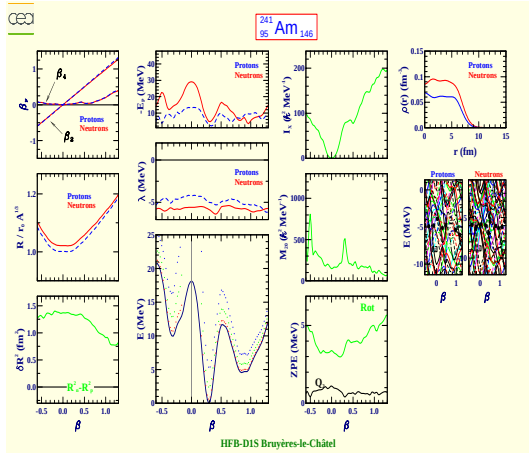
Americium 241 (Z=95, N=146)
