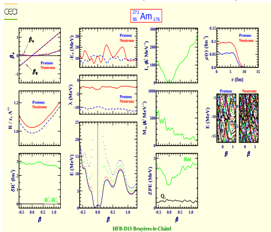
Americium 271 (Z=95, N=176)
