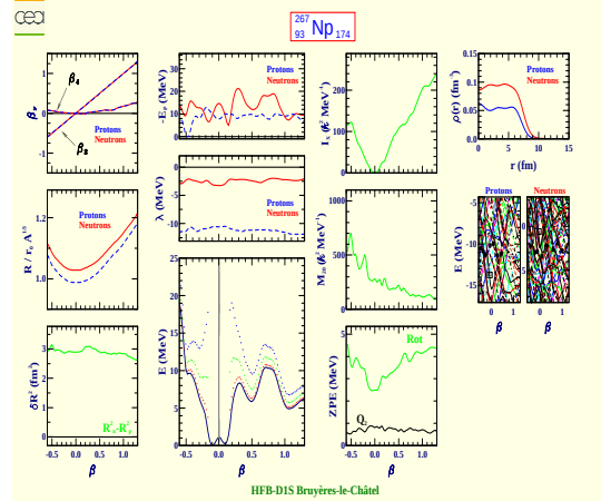
Neptunium 267 (Z=93, N=174)
