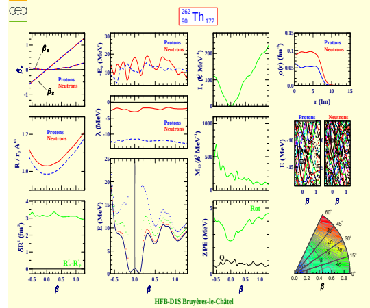
Thorium 262 (Z=90, N=172)
