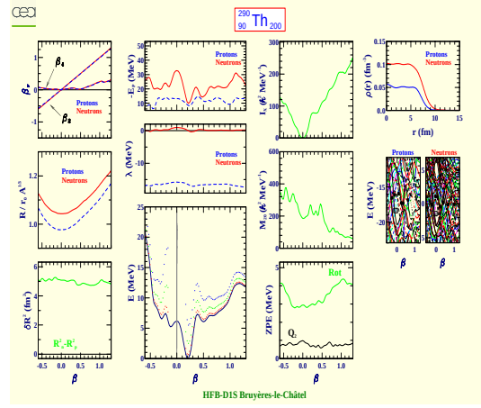
Thorium 290 (Z=90, N=200)
