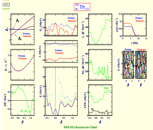
Thorium 207 (Z=90, N=117)
