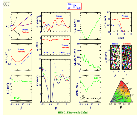
Thorium 268 (Z=90, N=178)
