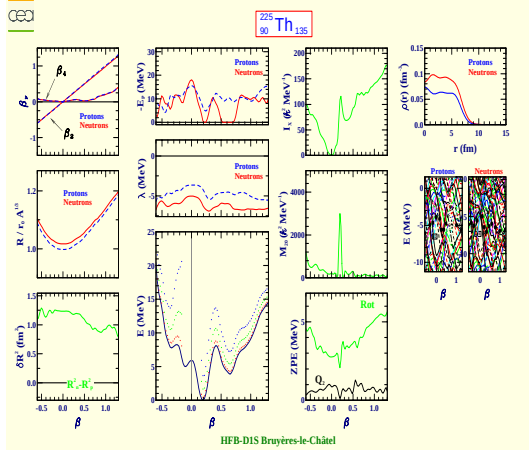
Thorium 225 (Z=90, N=135)
