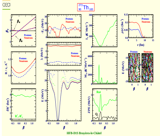
Thorium 273 (Z=90, N=183)
