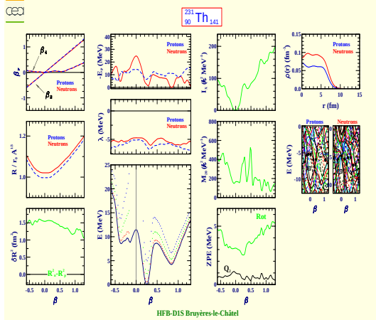
Thorium 231 (Z=90, N=141)
