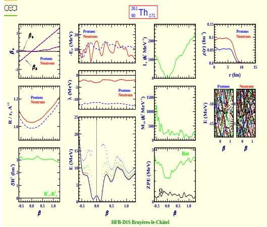
Thorium 261 (Z=90, N=171)
