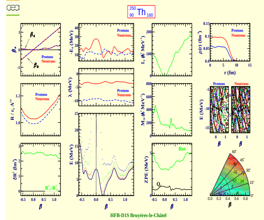
Thorium 250 (Z=90, N=160)
