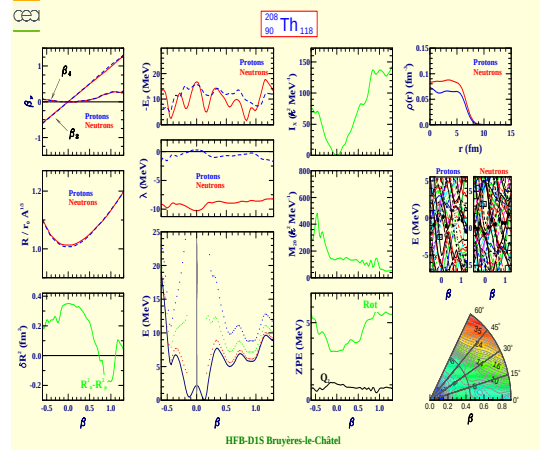
Thorium 208 (Z=90, N=118)
