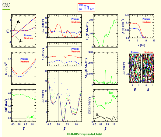
Thorium 237 (Z=90, N=147)
