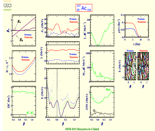
Actinium 247 (Z=89, N=158)
