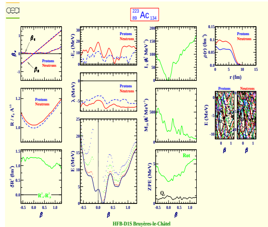
Actinium 223 (Z=89, N=134)
