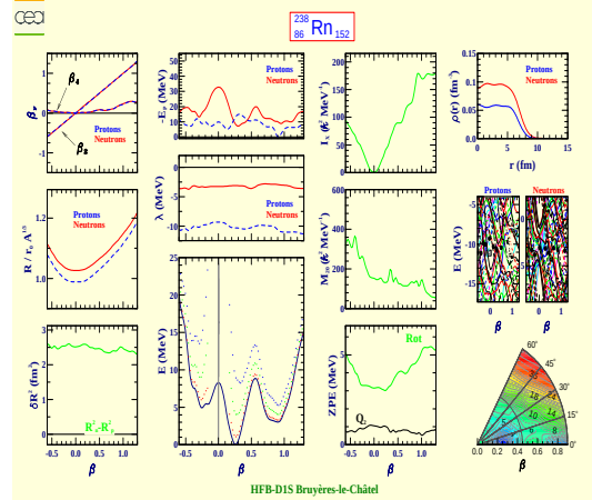
Radon 238 (Z=86, N=152)
