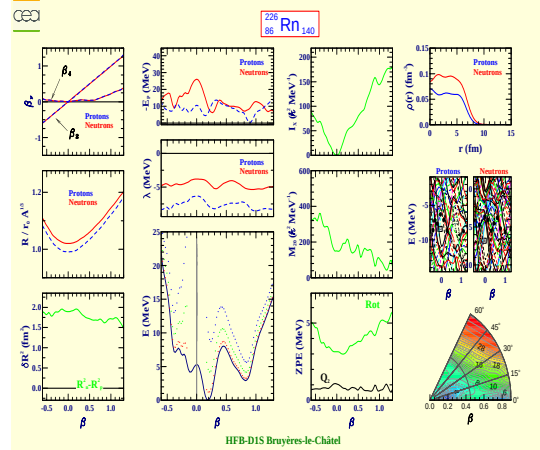
Radon 226 (Z=86, N=140)
