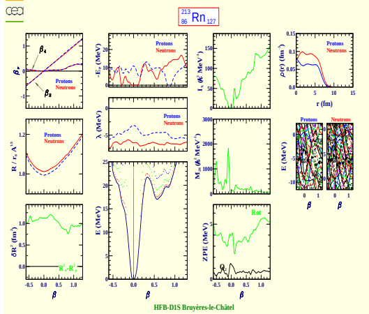
Radon 213 (Z=86, N=127)
