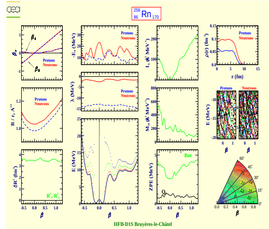
Radon 256 (Z=86, N=170)
