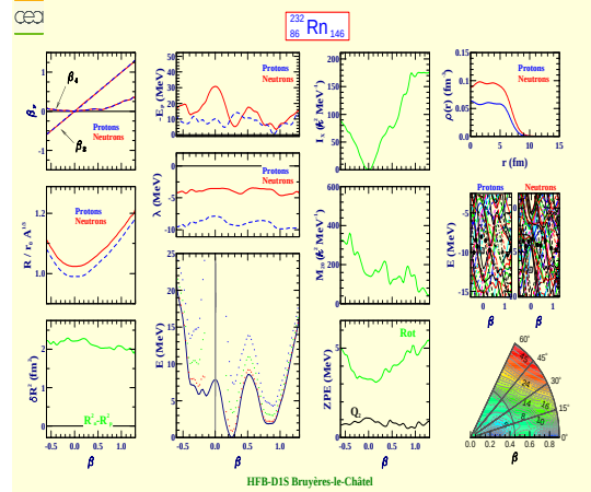
Radon 232 (Z=86, N=146)
