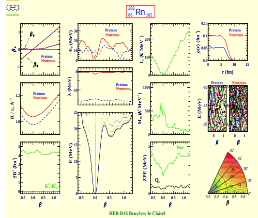
Radon 268 (Z=86, N=182)
