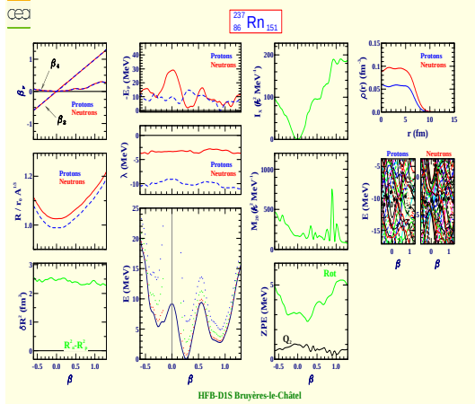
Radon 237 (Z=86, N=151)
