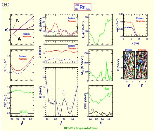
Radon 231 (Z=86, N=145)
