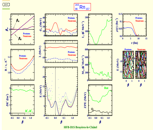
Radon 243 (Z=86, N=157)
