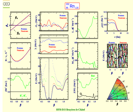
Radon 202 (Z=86, N=116)
