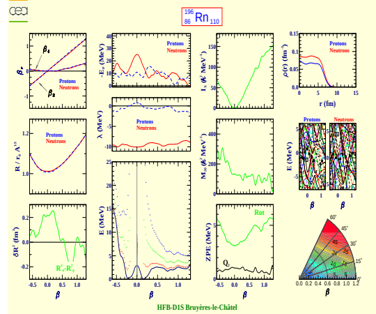
Radon 196 (Z=86, N=110)
