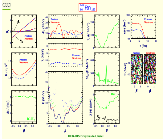
Radon 249 (Z=86, N=163)
