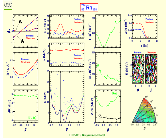
Radon 244 (Z=86, N=158)
