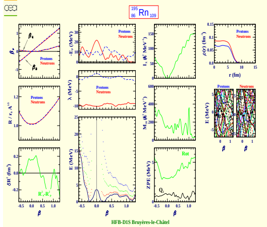
Radon 195 (Z=86, N=109)
