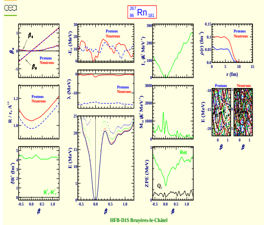
Radon 267 (Z=86, N=181)
