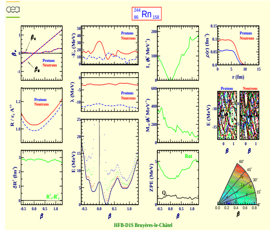
Radon 244 (Z=86, N=158)
