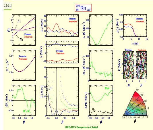
Radon 196 (Z=86, N=110)
