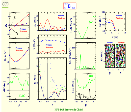
Bismuth 192 (Z=83, N=109)
