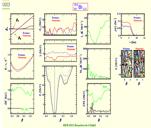
Bismuth 204 (Z=83, N=121)
