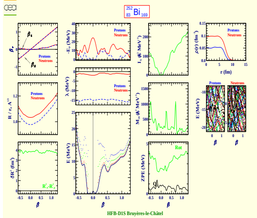
Bismuth 252 (Z=83, N=169)
