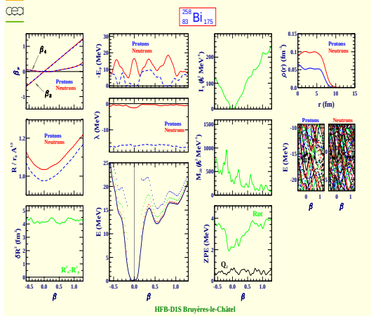
Bismuth 258 (Z=83, N=175)
