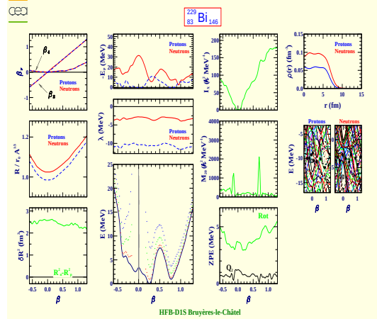
Bismuth 229 (Z=83, N=146)
