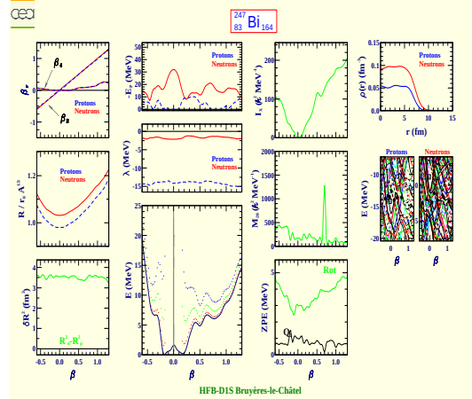
Bismuth 247 (Z=83, N=164)
