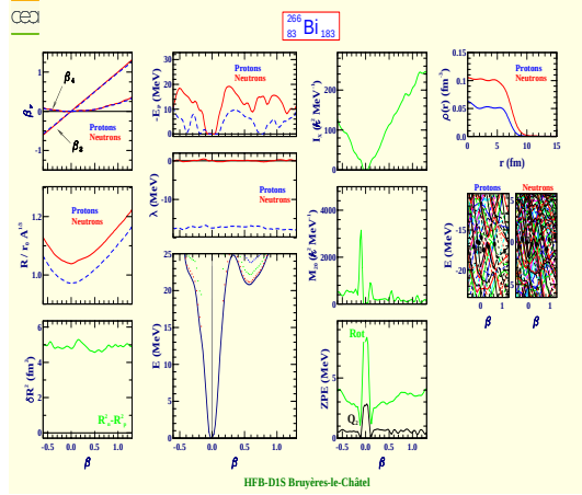
Bismuth 266 (Z=83, N=183)
