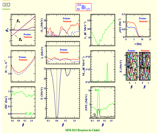
Bismuth 210 (Z=83, N=127)
