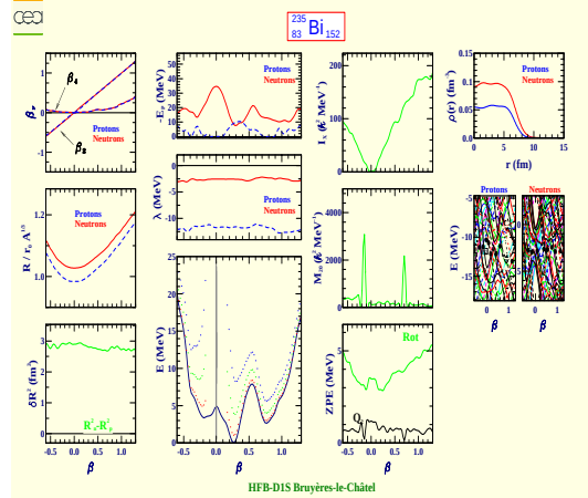
Bismuth 235 (Z=83, N=152)
