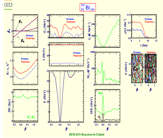
Bismuth 267 (Z=83, N=184)
