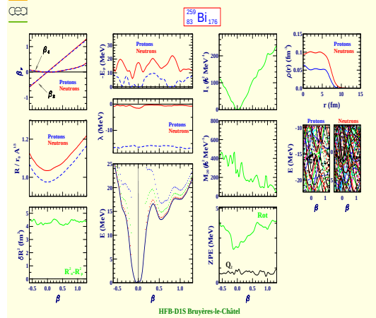
Bismuth 259 (Z=83, N=176)
