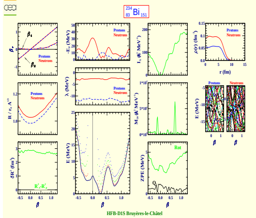
Bismuth 234 (Z=83, N=151)
