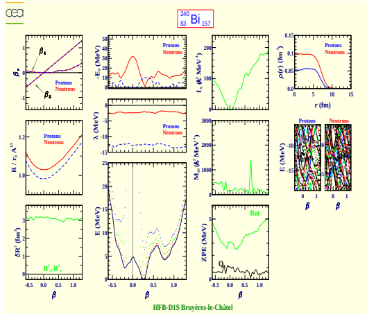
Bismuth 240 (Z=83, N=157)
