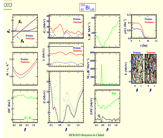
Bismuth 223 (Z=83, N=140)
