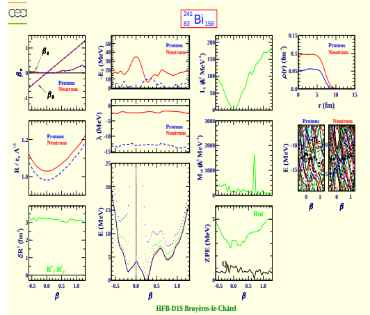
Bismuth 241 (Z=83, N=158)
