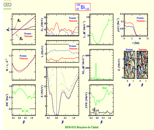
Bismuth 199 (Z=83, N=116)
