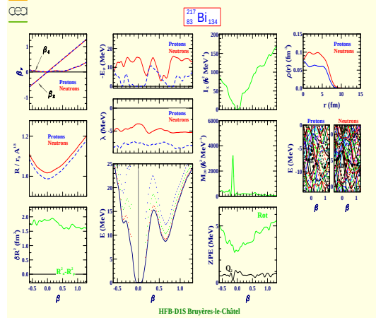
Bismuth 217 (Z=83, N=134)
