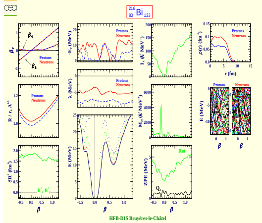
Bismuth 216 (Z=83, N=133)
