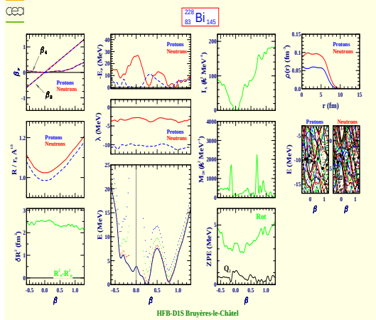
Bismuth 228 (Z=83, N=145)
