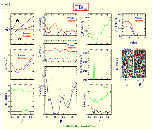
Bismuth 222 (Z=83, N=139)
