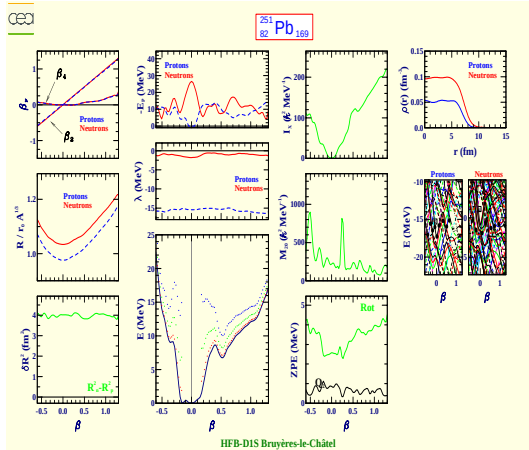
Plomb 251 (Z=82, N=169)
