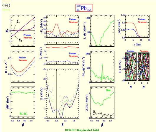
Plomb 239 (Z=82, N=157)
