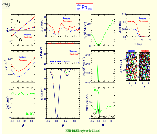
Plomb 265 (Z=82, N=183)
