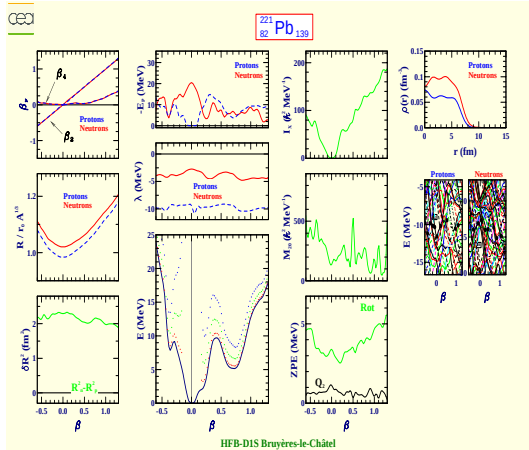
Plomb 221 (Z=82, N=139)
