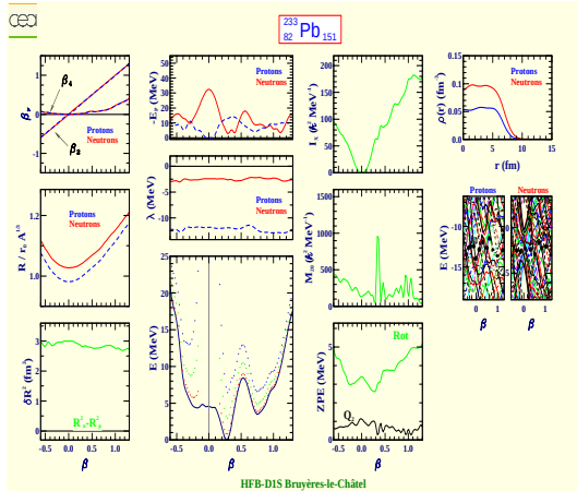
Plomb 233 (Z=82, N=151)
