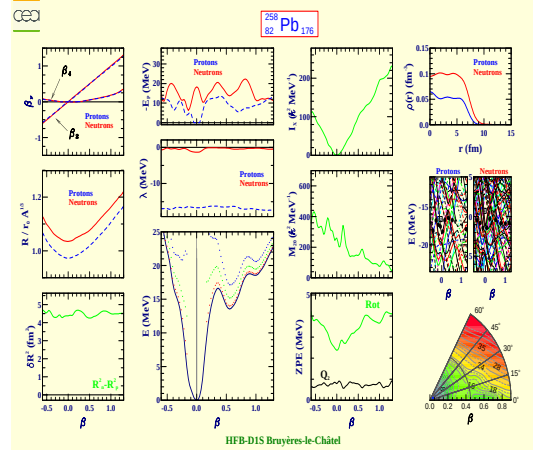
Plomb 258 (Z=82, N=176)
