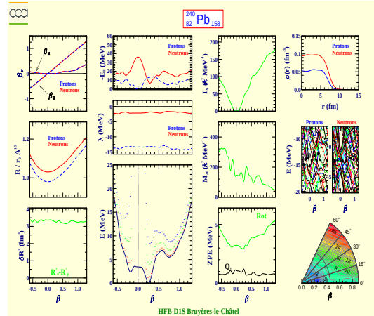
Plomb 240 (Z=82, N=158)
