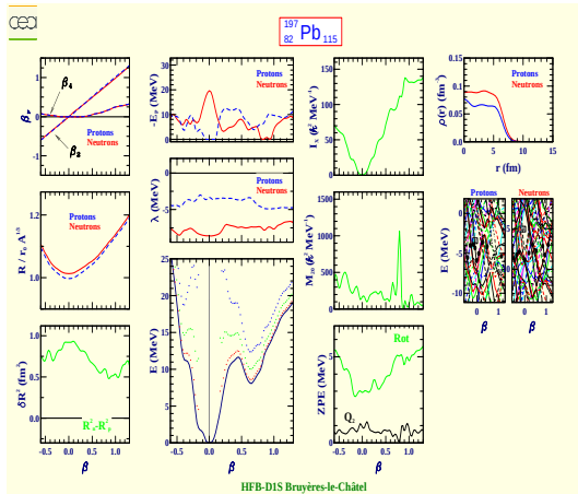
Plomb 197 (Z=82, N=115)
