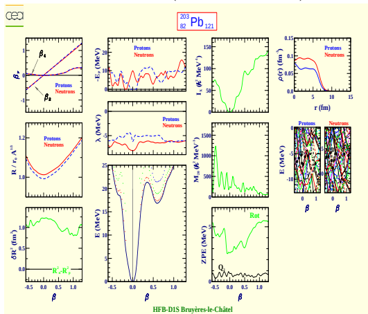
Plomb 203 (Z=82, N=121)
