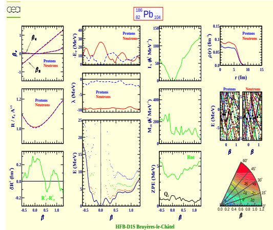
Plomb 186 (Z=82, N=104)
