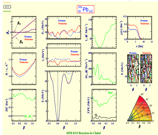
Plomb 204 (Z=82, N=122)
