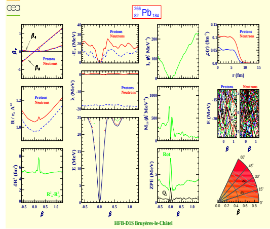
Plomb 266 (Z=82, N=184)
