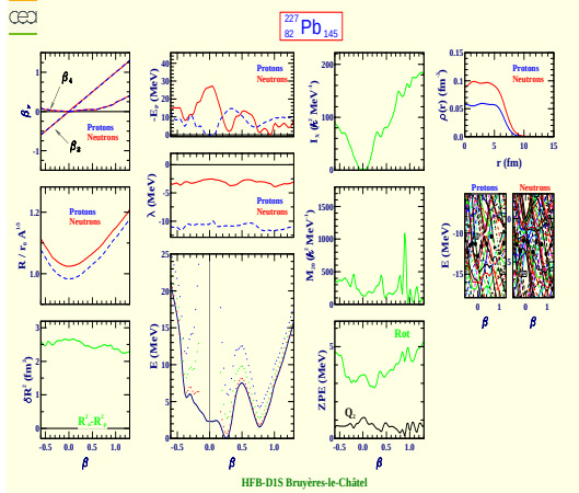
Plomb 227 (Z=82, N=145)
