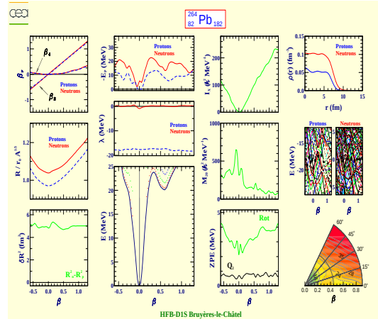
Plomb 264 (Z=82, N=182)
