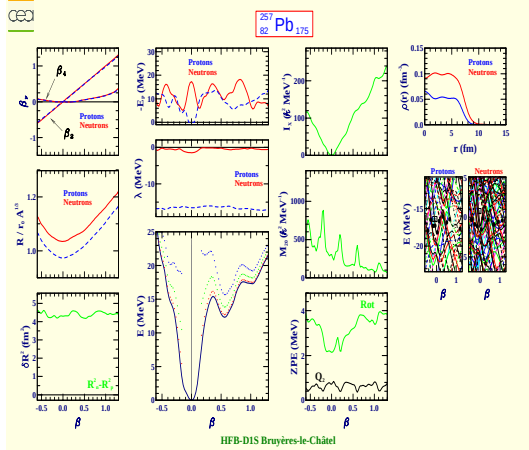
Plomb 257 (Z=82, N=175)
