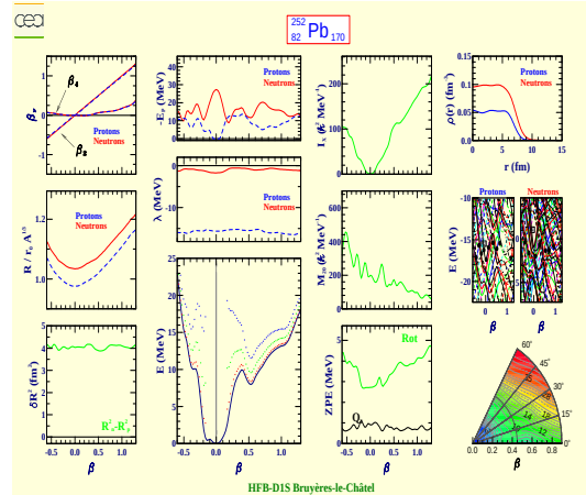
Plomb 252 (Z=82, N=170)
