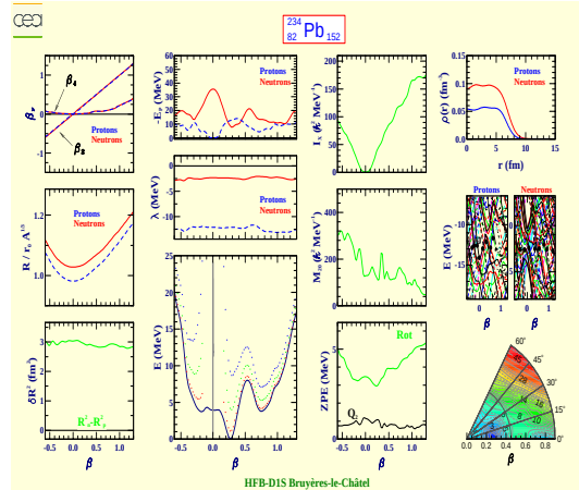
Plomb 234 (Z=82, N=152)
