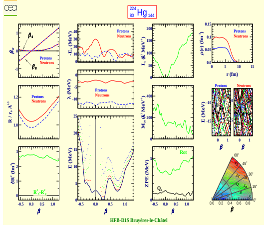
Mercure 224 (Z=80, N=144)
