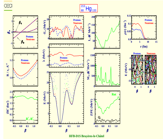
Mercure 213 (Z=80, N=133)
