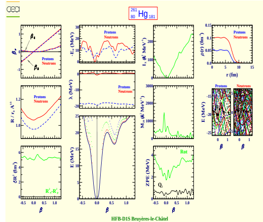
Mercure 261 (Z=80, N=181)
