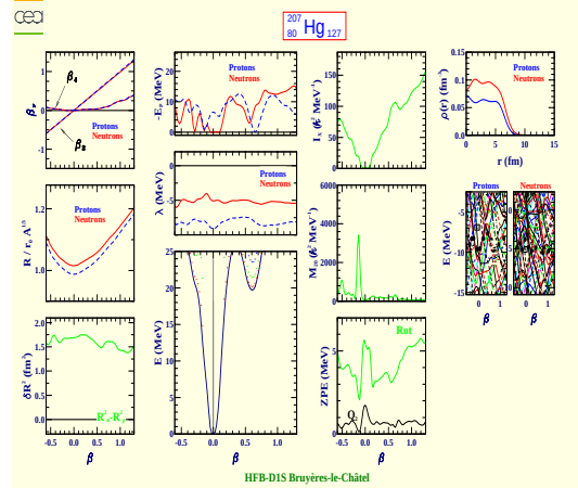
Mercure 207 (Z=80, N=127)
