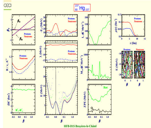
Mercure 237 (Z=80, N=157)
