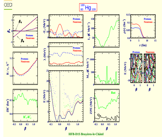
Mercure 189 (Z=80, N=109)
