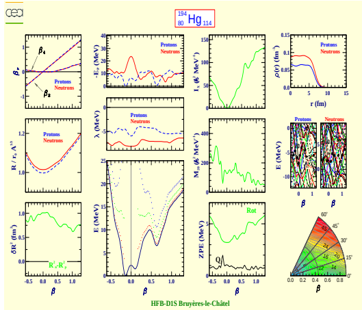
Mercure 194 (Z=80, N=114)
