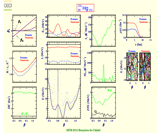
Mercure 231 (Z=80, N=151)
