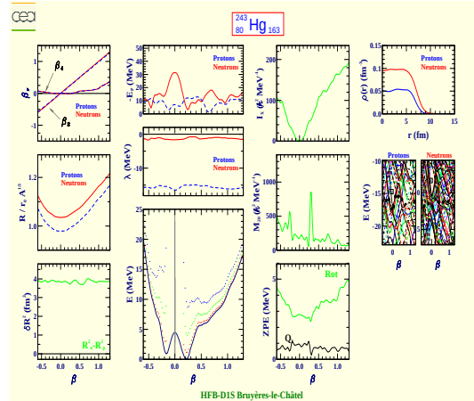
Mercure 243 (Z=80, N=163)
