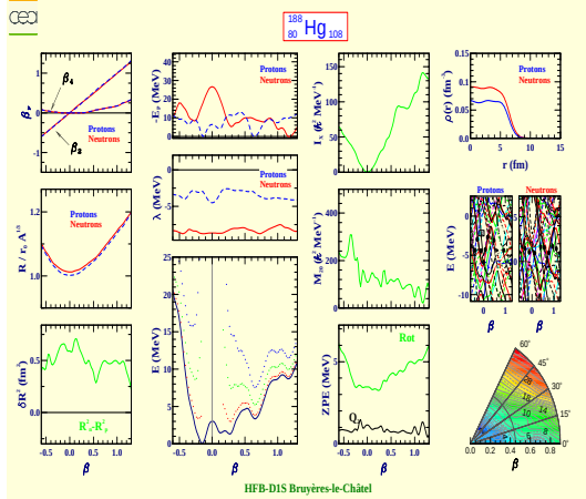
Mercure 188 (Z=80, N=108)
