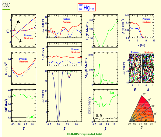
Mercure 206 (Z=80, N=126)
