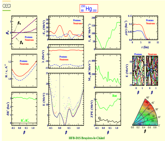
Mercure 230 (Z=80, N=150)
