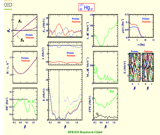
Mercure 177 (Z=80, N=97)
