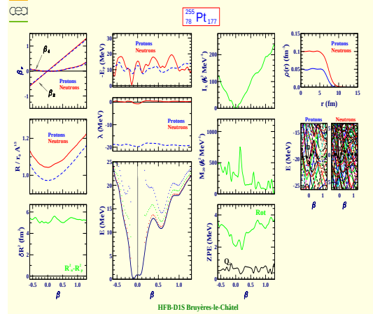
Platinum 255 (Z=78, N=177)
