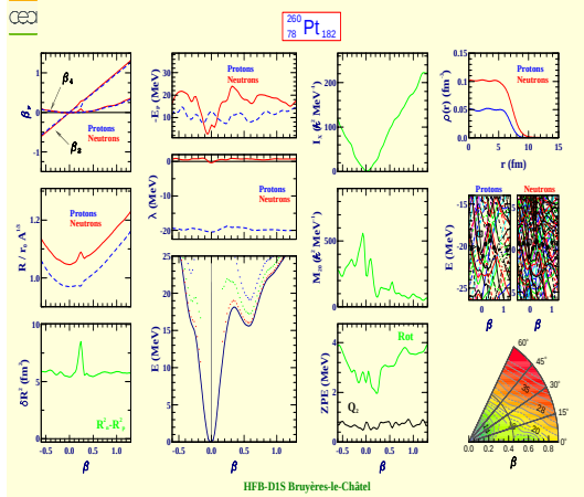
Platinum 260 (Z=78, N=182)
