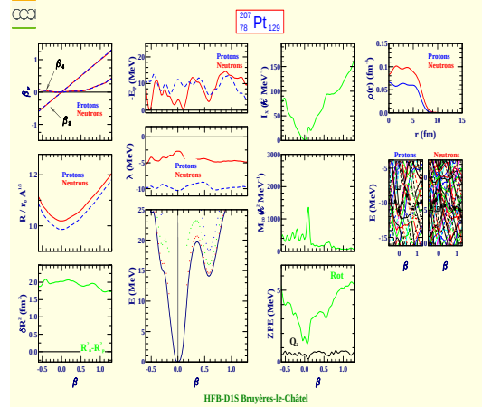
Platinum 207 (Z=78, N=129)
