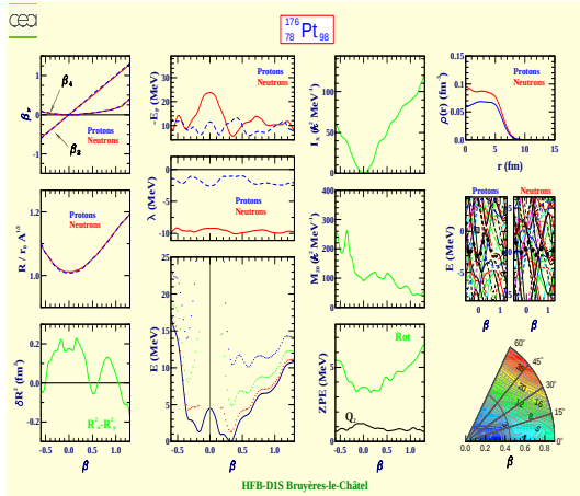
Platinum 176 (Z=78, N=98)
