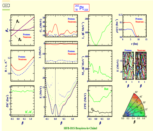
Platinum 242 (Z=78, N=164)
