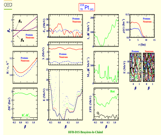
Platinum 219 (Z=78, N=141)
