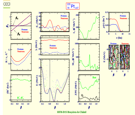
Platinum 225 (Z=78, N=147)
