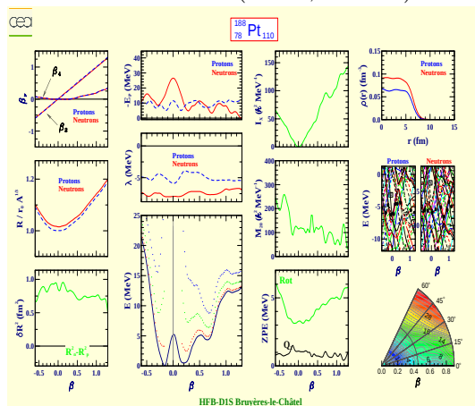
Platinum 188 (Z=78, N=110)
