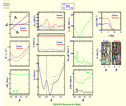
Platine 237 (Z=78, N=159)
