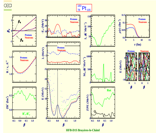
Platine 183 (Z=78, N=105)
