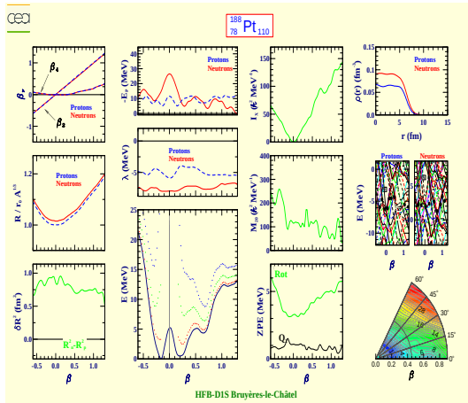
Platine 188 (Z=78, N=110)
