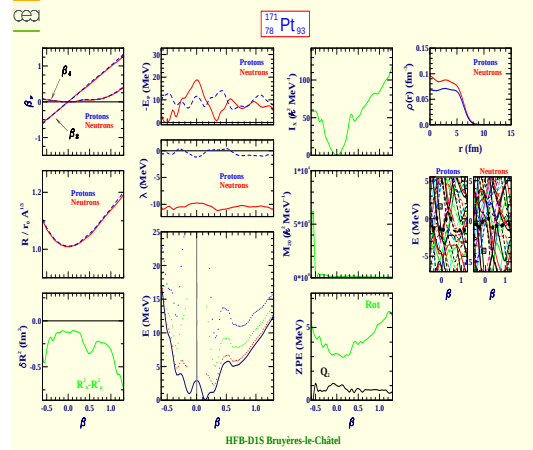
Platine 171 (Z=78, N=93)
