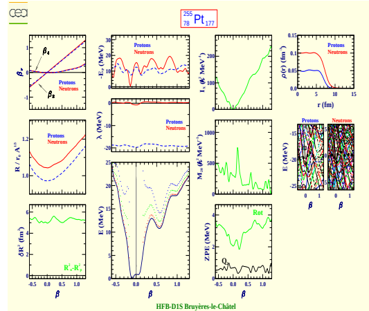
Platine 255 (Z=78, N=177)
