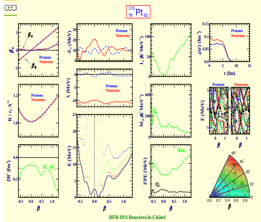
Platine 170 (Z=78, N=92)
