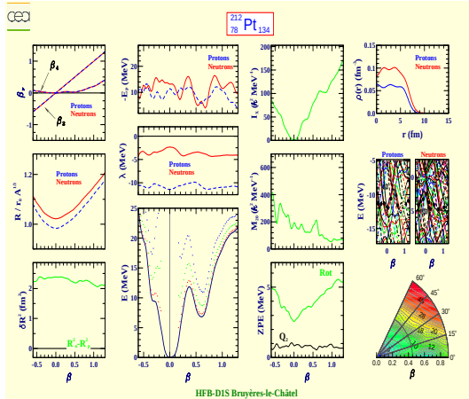
Platine 212 (Z=78, N=134)
