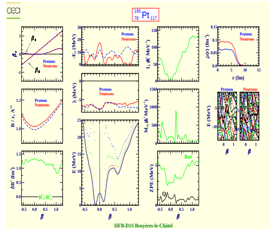
Platine 195 (Z=78, N=117)
