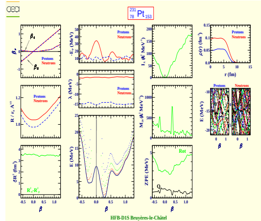
Platine 231 (Z=78, N=153)
