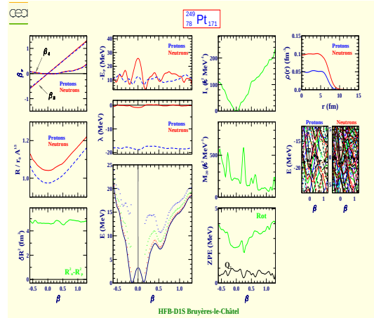
Platine 249 (Z=78, N=171)
