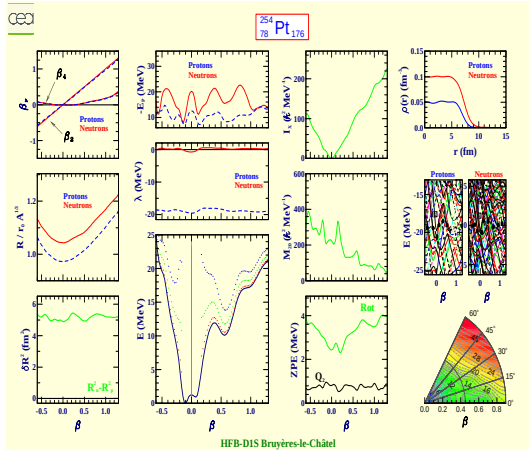
Platine 254 (Z=78, N=176)
