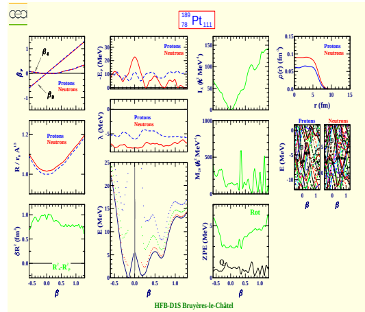
Platine 189 (Z=78, N=111)
