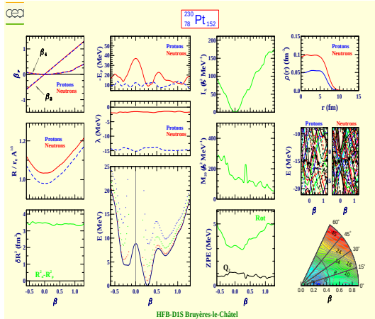
Platine 230 (Z=78, N=152)
