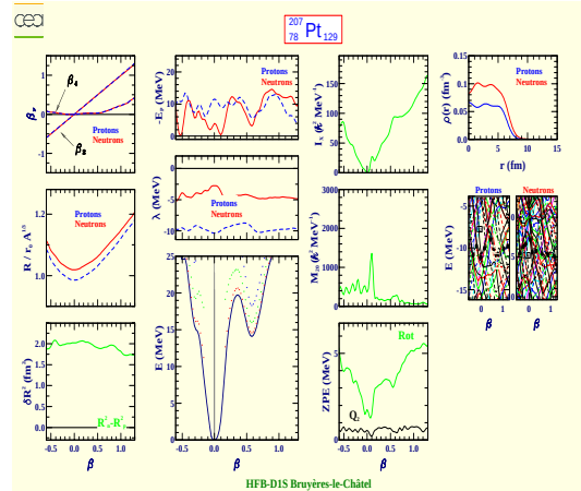
Platine 207 (Z=78, N=129)
