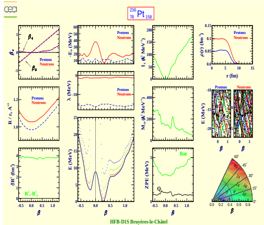
Platine 236 (Z=78, N=158)
