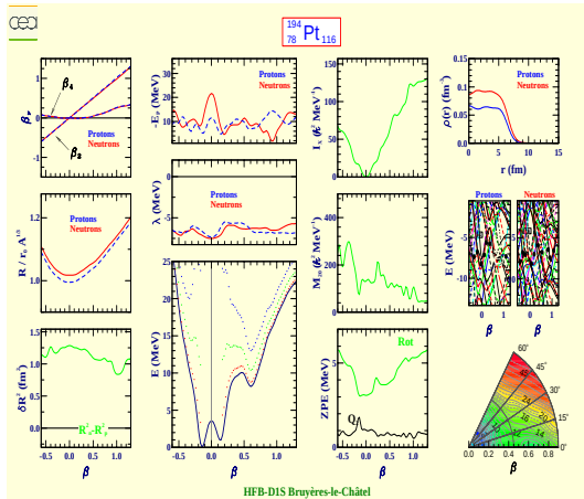
Platine 194 (Z=78, N=116)
