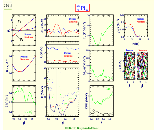
Platine 177 (Z=78, N=99)
