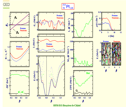
Platine 213 (Z=78, N=135)
