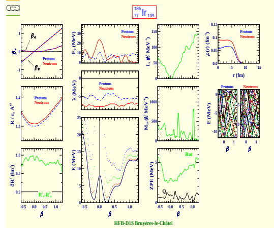
Iridium 186 (Z=77, N=109)
