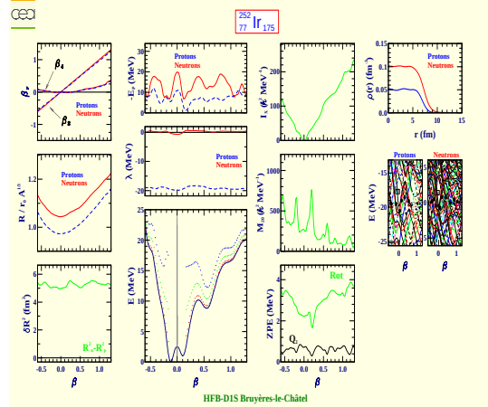
Iridium 252 (Z=77, N=175)
