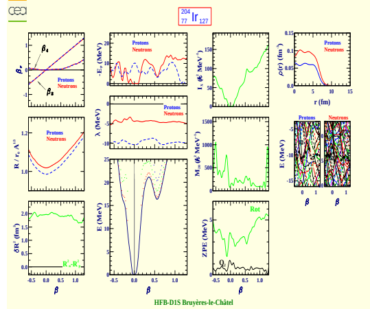
Iridium 204 (Z=77, N=127)
