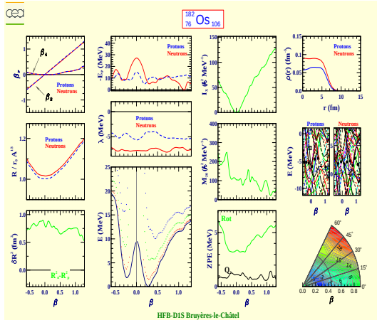
Osmium 182 (Z=76, N=106)
