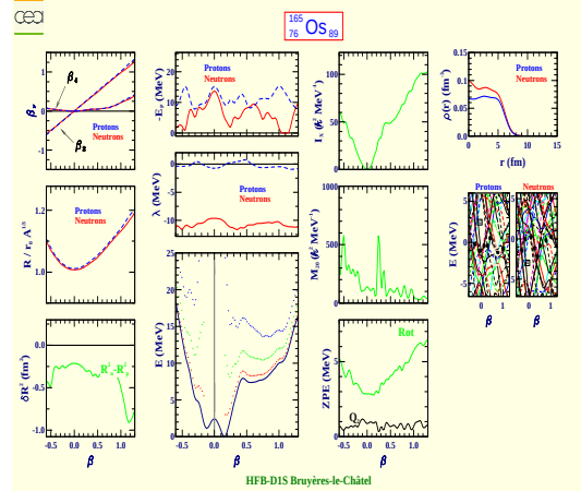
Osmium 165 (Z=76, N=89)
