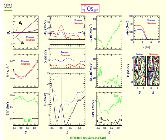
Osmium 183 (Z=76, N=107)
