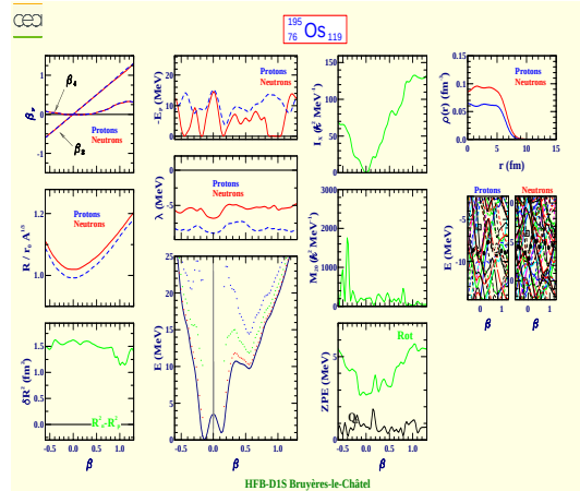
Osmium 195 (Z=76, N=119)
