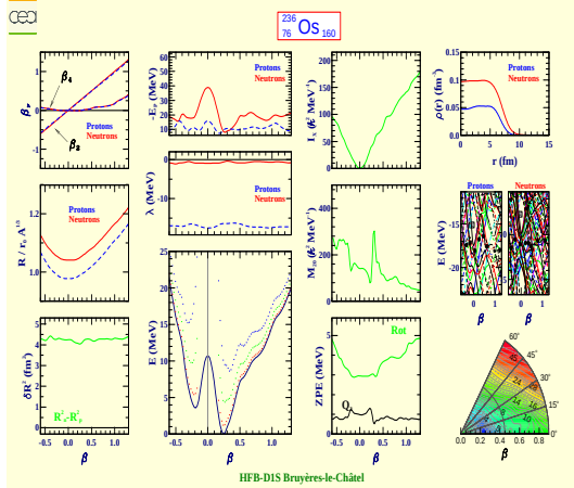
Osmium 236 (Z=76, N=160)
