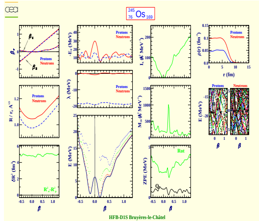
Osmium 245 (Z=76, N=169)
