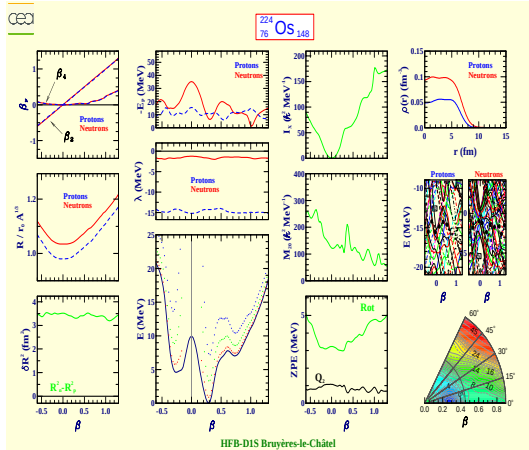
Osmium 224 (Z=76, N=148)
