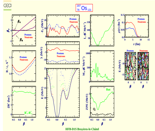
Osmium 207 (Z=76, N=131)
