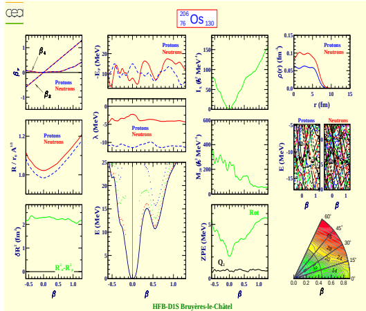
Osmium 206 (Z=76, N=130)
