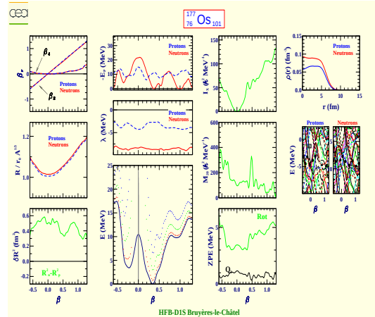
Osmium 177 (Z=76, N=101)
