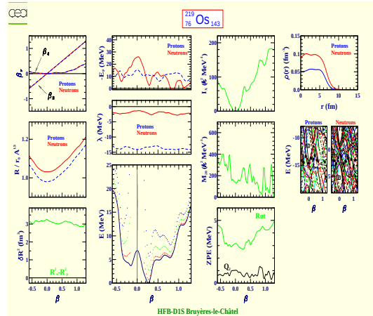
Osmium 219 (Z=76, N=143)
