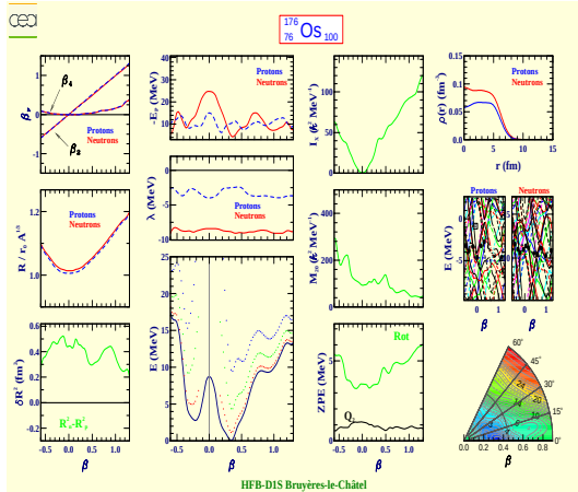
Osmium 176 (Z=76, N=100)
