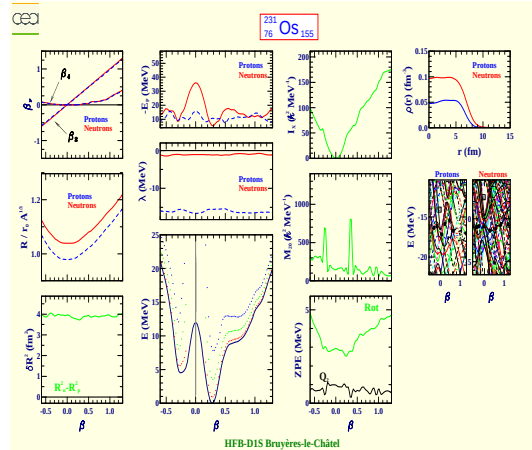
Osmium 231 (Z=76, N=155)
