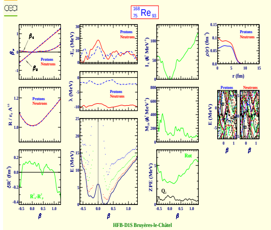
Rhenium 168 (Z=75, N=93)
