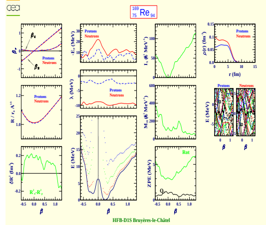
Rhenium 169 (Z=75, N=94)
