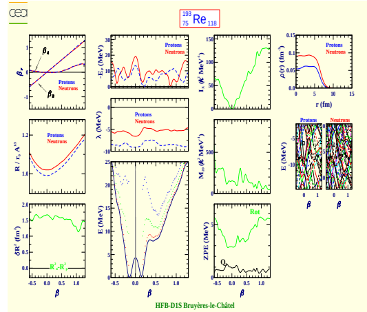
Rhenium 193 (Z=75, N=118)
