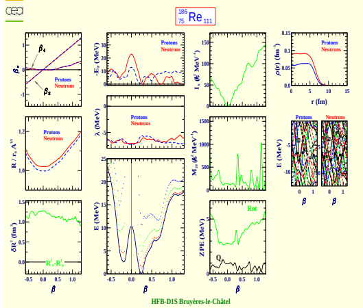
Rhenium 186 (Z=75, N=111)
