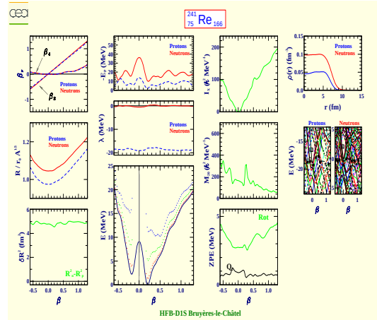
Rhenium 241 (Z=75, N=166)
