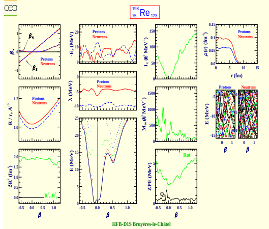
Rhenium 198 (Z=75, N=123)
