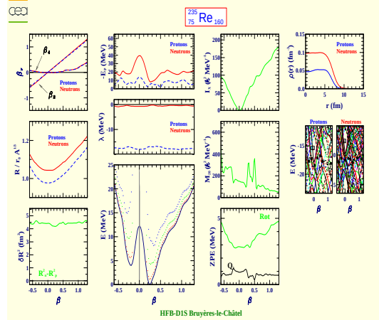
Rhenium 235 (Z=75, N=160)
