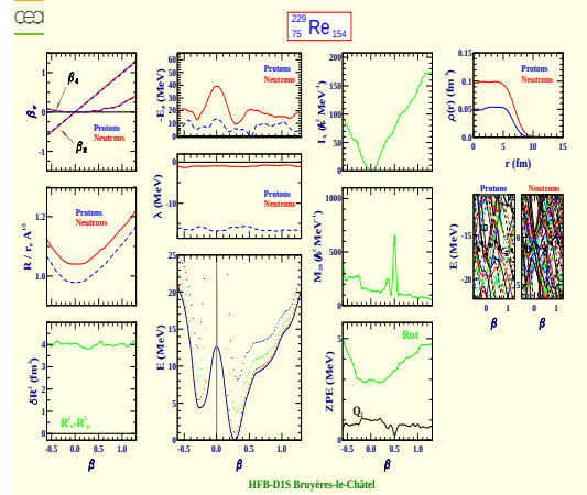
Rhenium 229 (Z=75, N=154)
