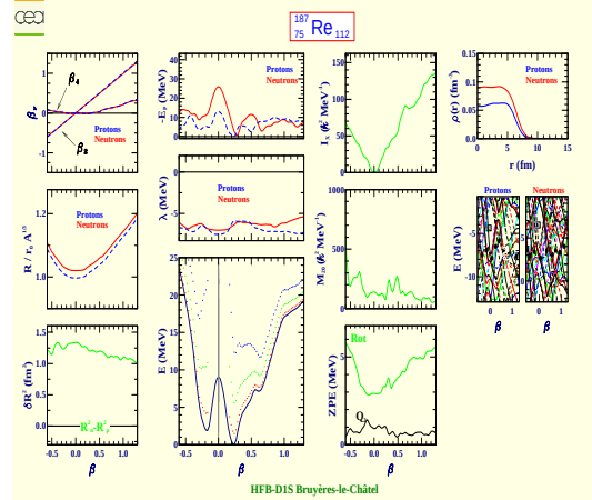
Rhenium 187 (Z=75, N=112)
