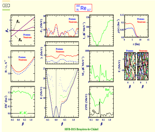
Rhenium 192 (Z=75, N=117)
