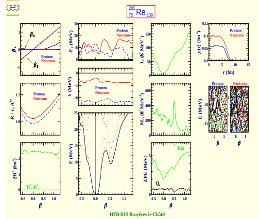
Rhenium 205 ( Z=75 , N=130 )
