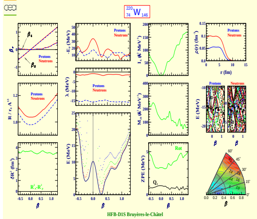
Tungsten 220 (Z=74, N=146)
