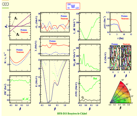
Tungsten 196 (Z=74, N=122)
