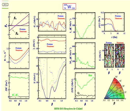
Tungsten 208 (Z=74, N=134)
