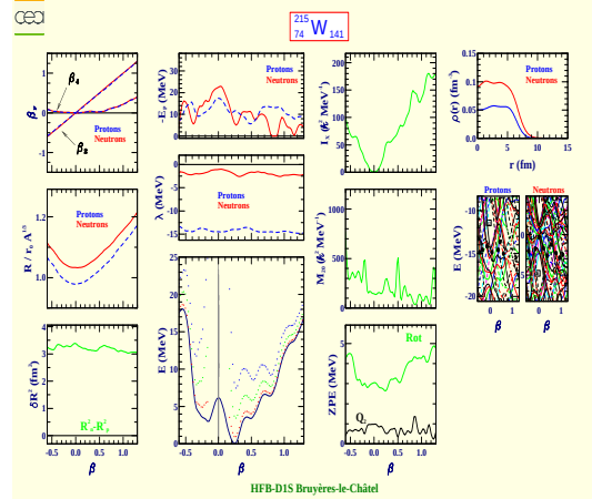
Tungsten 215 (Z=74, N=141)
