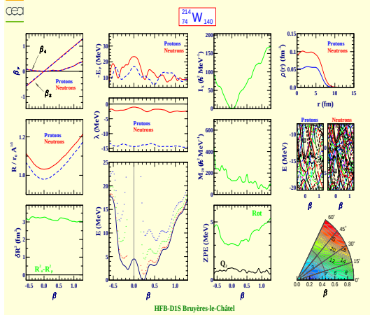
Tungsten 214 (Z=74, N=140)
