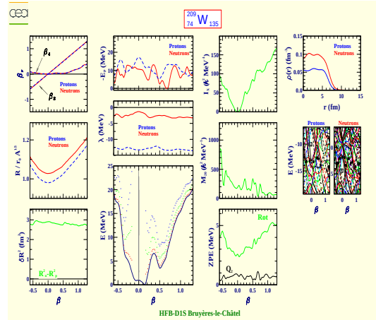
Tungsten 209 (Z=74, N=135)
