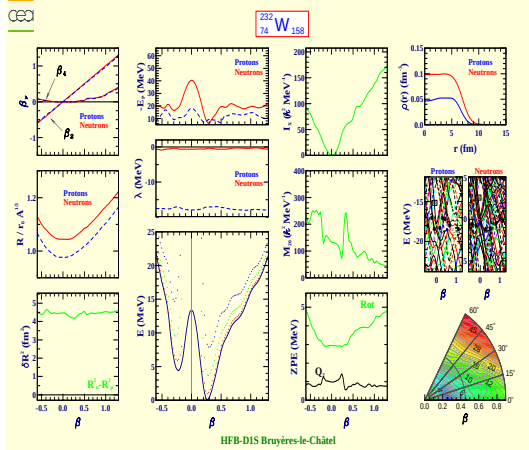
Tungsten 232 (Z=74, N=158)
