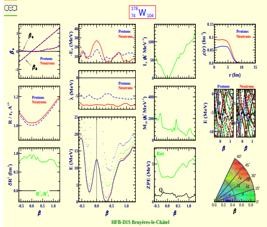
Tungsten 178 (Z=74, N=104)
