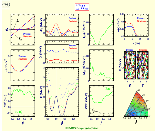
Tungsten 172 (Z=74, N=98)
