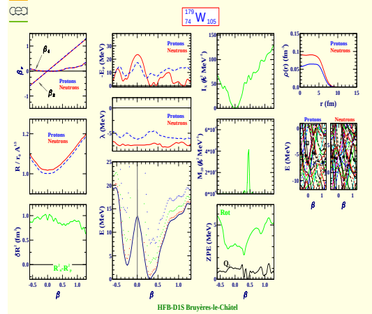
Tungsten 179 (Z=74, N=105)
