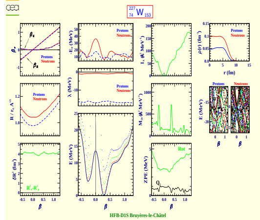
Tungsten 227 (Z=74, N=153)
