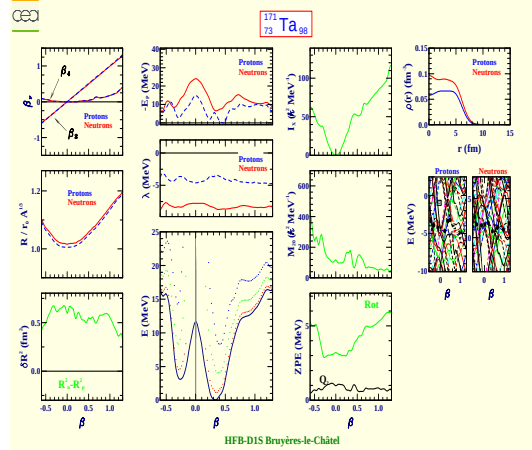
Tantalum 171 (Z=73, N=98)
