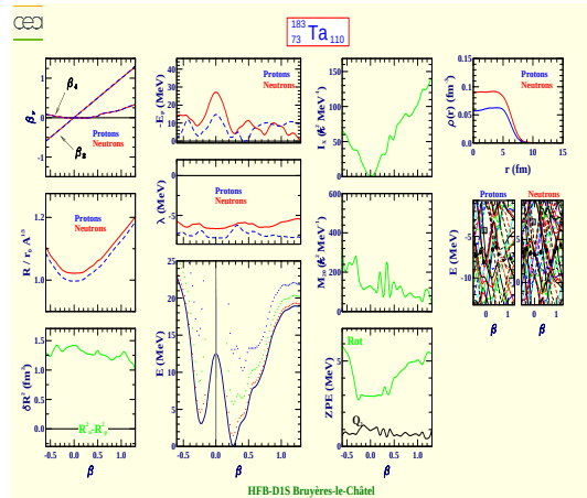
Tantalum 183 (Z=73, N=110)
