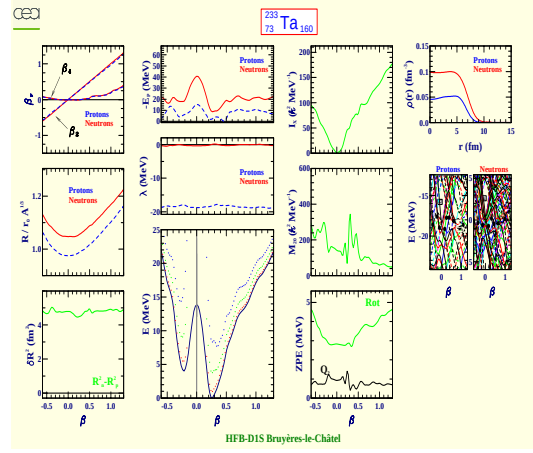
Tantalum 233 (Z=73, N=160)
