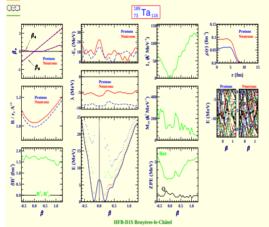
Tantalum 189 (Z=73, N=116)
