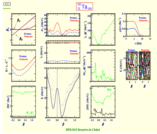
Tantalum 232 (Z=73, N=159)
