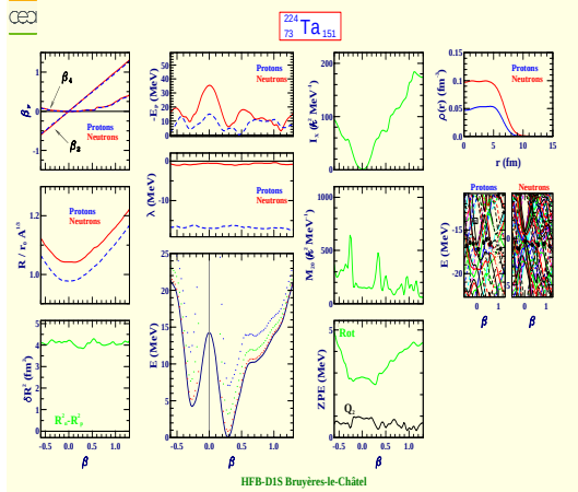
Tantalum 224 (Z=73, N=151)
