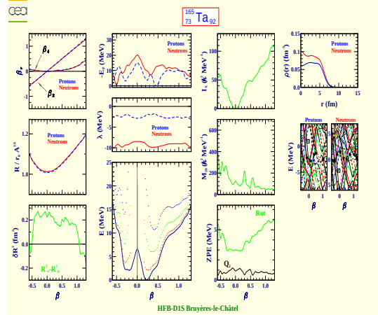
Tantalum 165 (Z=73, N=92)
