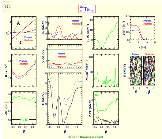
Tantalum 182 (Z=73, N=109)
