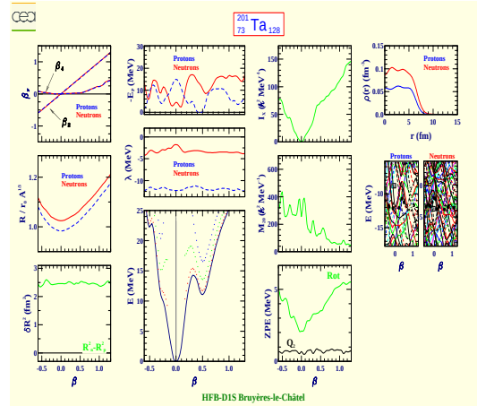
Tantalum 201 (Z=73, N=128)
