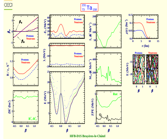
Tantalum 231 (Z=73, N=158)
