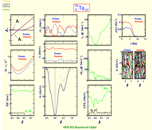
Tantalum 200 (Z=73, N=127)
