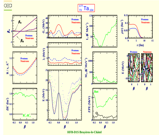
Tantalum 177 (Z=73, N=104)
