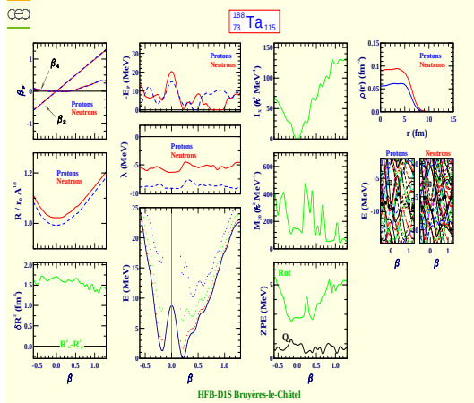
Tantalum 188 (Z=73, N=115)
