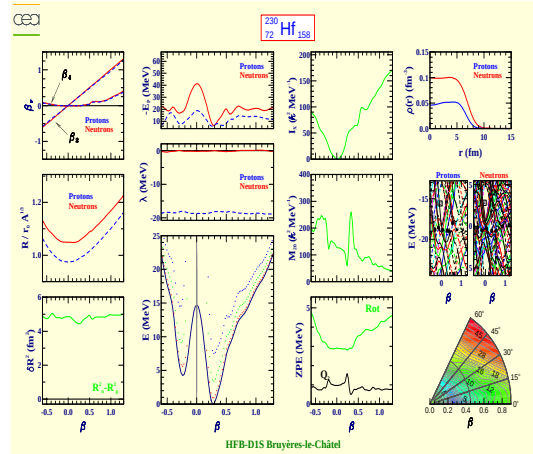
Hafnium 230 (Z=72, N=158)
