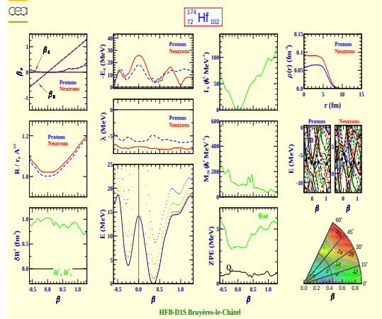
Hafnium 174 (Z=72, N=102)
