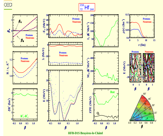
Hafnium 216 (Z=72, N=144)
