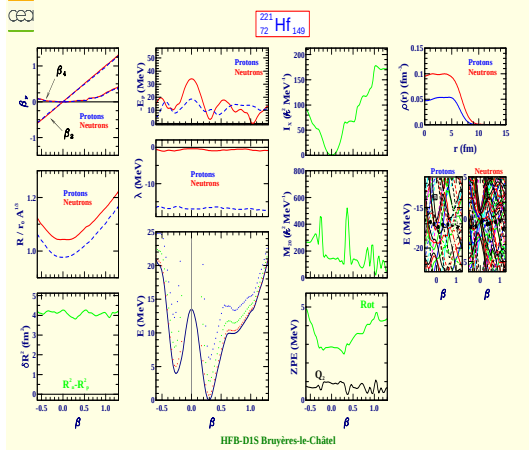
Hafnium 221 (Z=72, N=149)
