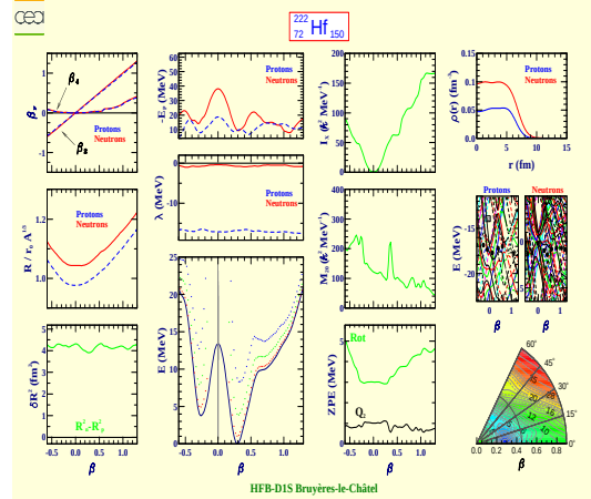
Hafnium 222 (Z=72, N=150)
