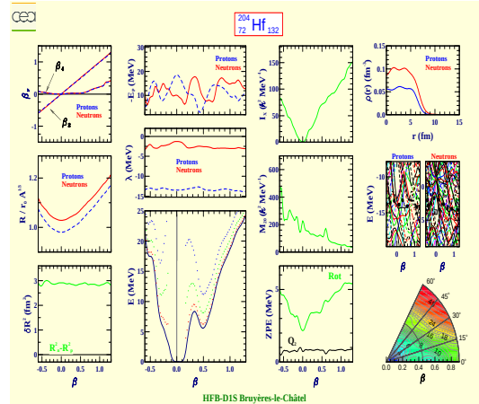
Hafnium 204 (Z=72, N=132)
