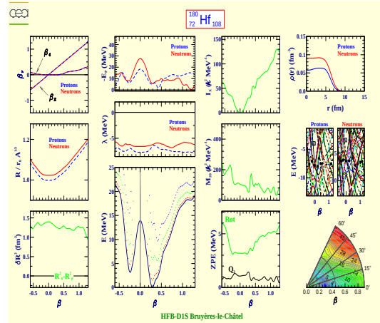
Hafnium 180 (Z=72, N=108)
