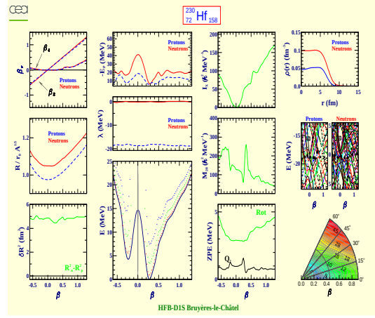
Hafnium 230 (Z=72, N=158)
