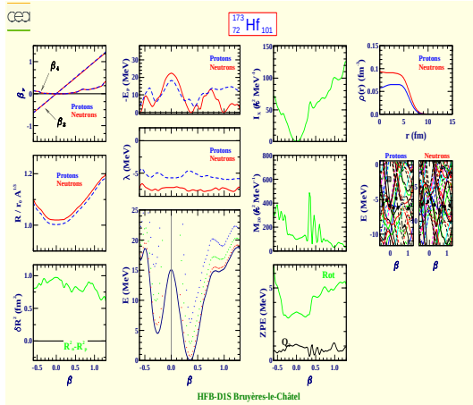
Hafnium 173 (Z=72, N=101)
