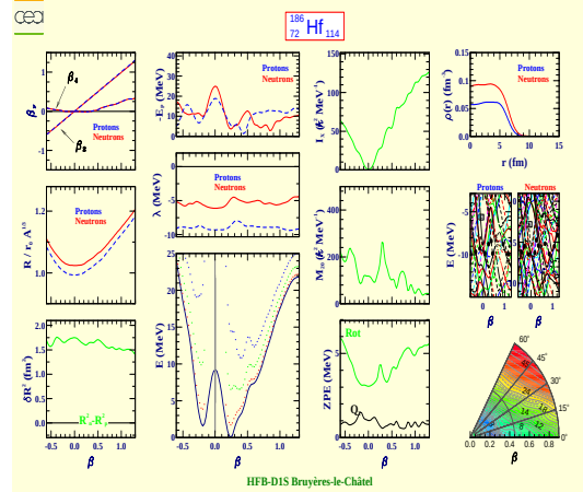
Hafnium 186 (Z=72, N=114)
