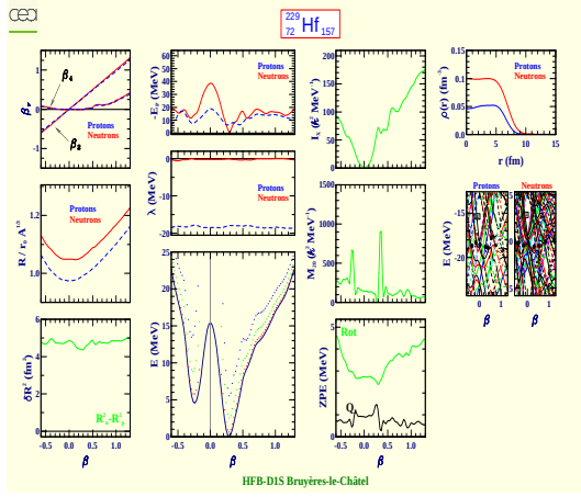
Hafnium 229 (Z=72, N=157)
