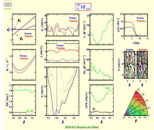
Hafnium 192 (Z=72, N=120)
