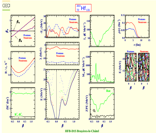
Hafnium 203 (Z=72, N=131)
