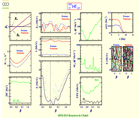
Hafnium 209 (Z=72, N=137)
