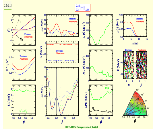
Hafnium 216 (Z=72, N=144)
