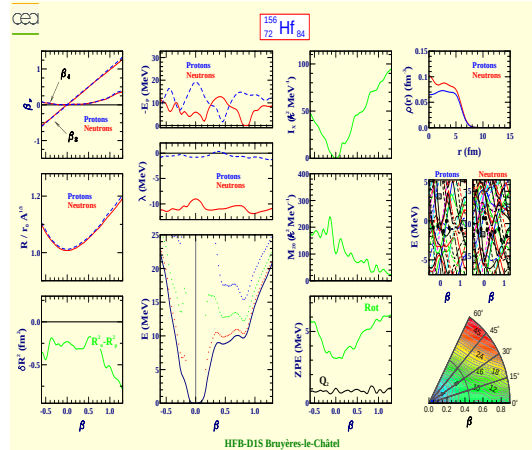
Hafnium 156 (Z=72, N=84)
