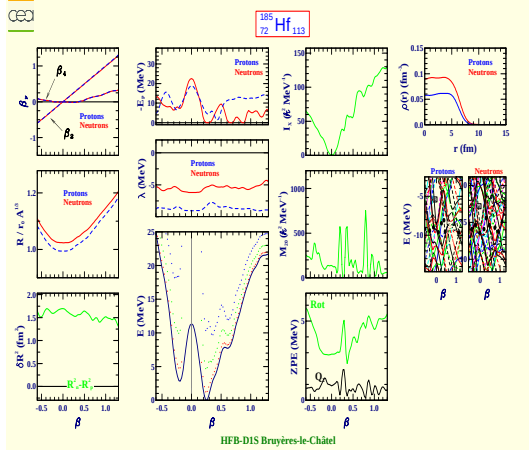
Hafnium 185 (Z=72, N=113)
