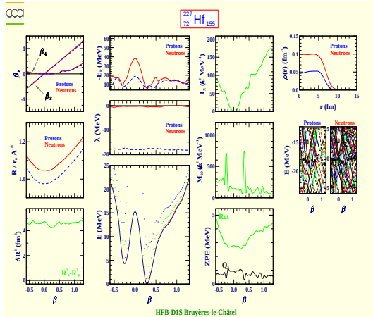
Hafnium 227 (Z=72, N=155)
