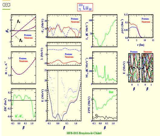
Lutetium 159 (Z=71, N=88)
