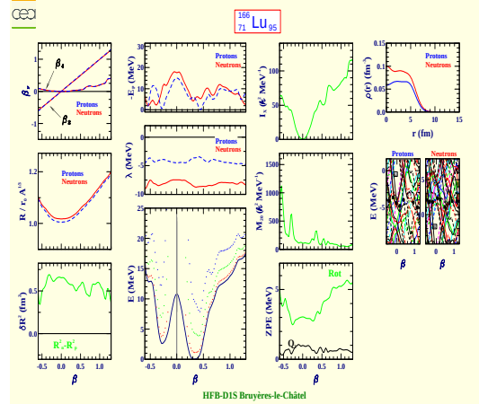
Lutetium 166 (Z=71, N=95)
