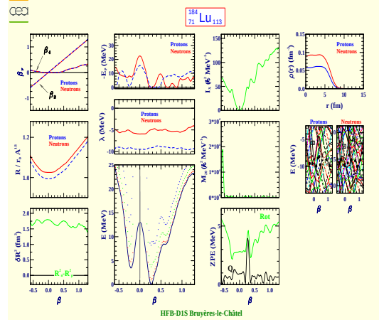
Lutetium 184 (Z=71, N=113)
