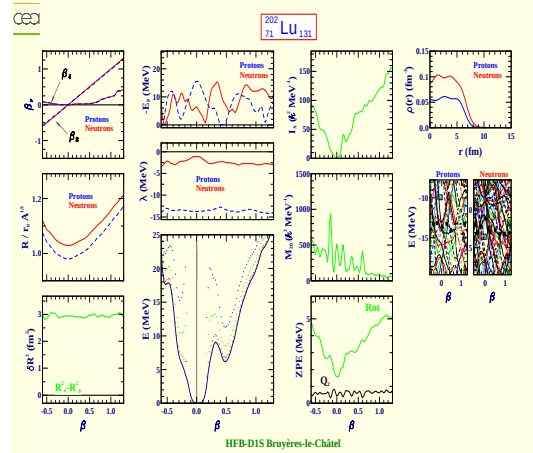
Lutetium 202 (Z=71, N=131)
