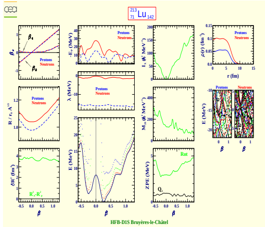
Lutetium 213 (Z=71, N=142)
