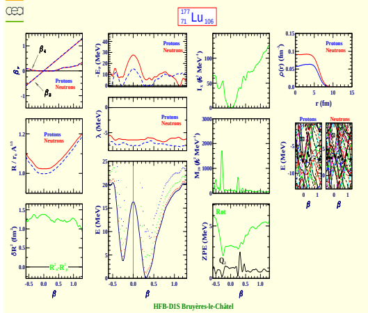
Lutetium 177 (Z=71, N=106)
