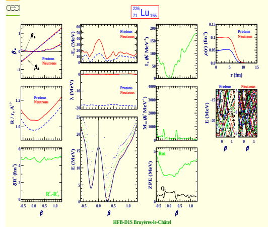
Lutetium 226 (Z=71, N=155)
