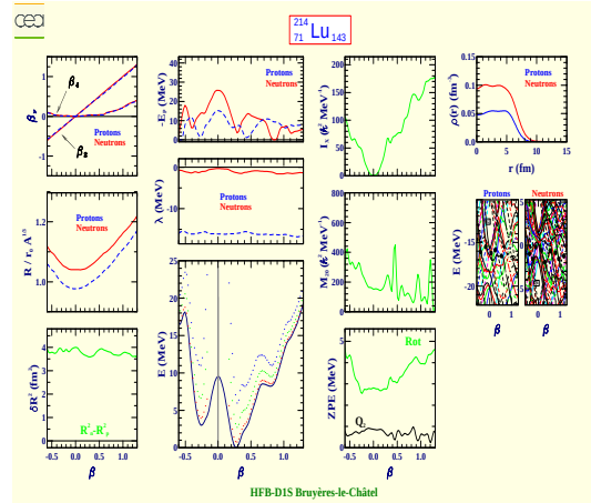
Lutetium 214 (Z=71, N=143)
