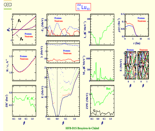
Lutetium 154 (Z=71, N=83)
