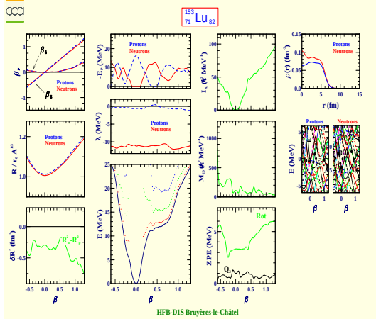
Lutetium 153 (Z=71, N=82)
