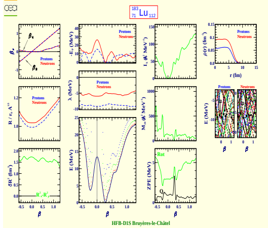
Lutetium 183 (Z=71, N=112)
