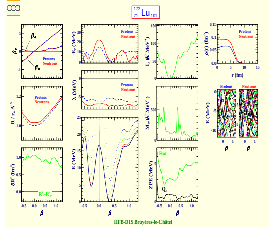
Lutetium 172 (Z=71, N=101)
