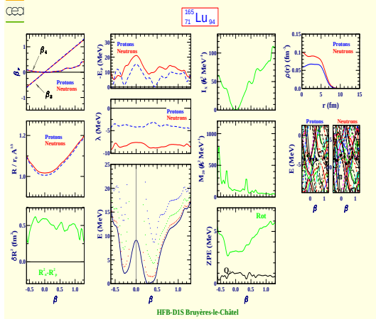
Lutetium 165 (Z=71, N=94)
