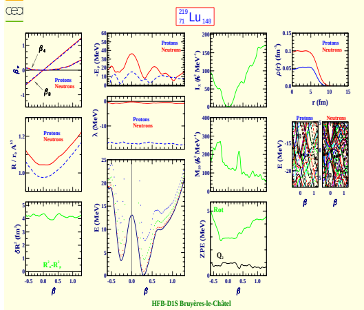
Lutetium 219 (Z=71, N=148)
