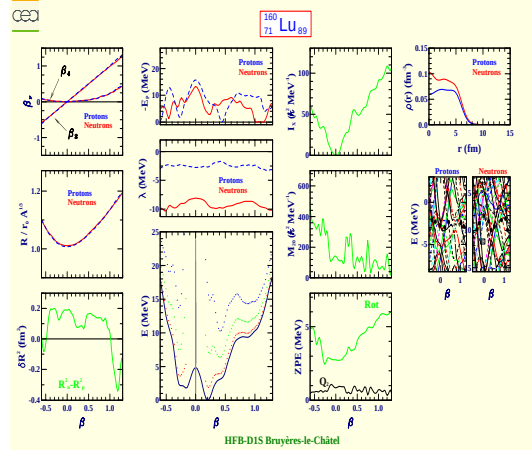
Lutetium 160 (Z=71, N=89)
