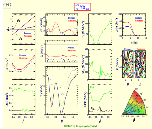
Ytterbium 176 (Z=70, N=106)
