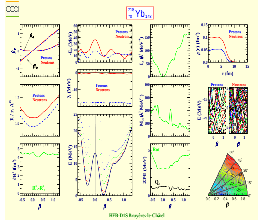
Ytterbium 218 (Z=70, N=148)
