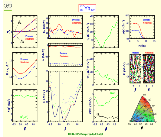
Ytterbium 212 (Z=70, N=142)
