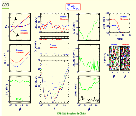
Ytterbium 211 (Z=70, N=141)
