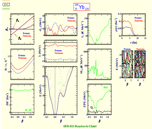
Ytterbium 199 (Z=70, N=129)
