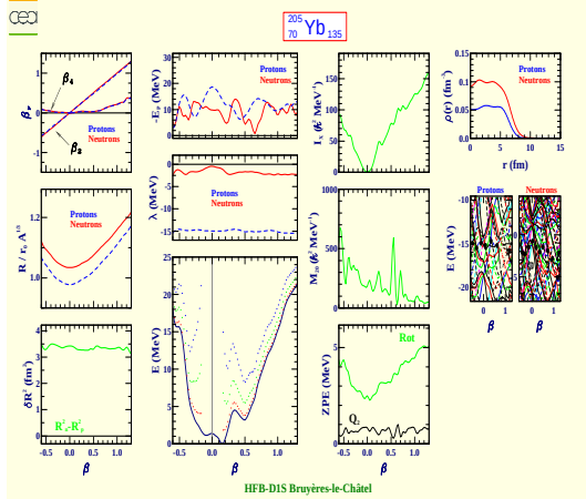
Ytterbium 205 (Z=70, N=135)
