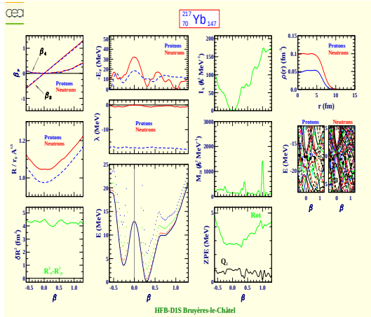
Ytterbium 217 (Z=70, N=147)
