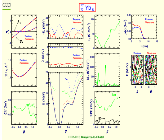
Ytterbium 151 (Z=70, N=81)
