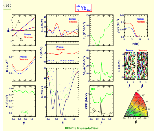
Ytterbium 182 (Z=70, N=112)
