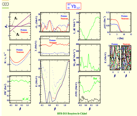
Ytterbium 187 (Z=70, N=117)
