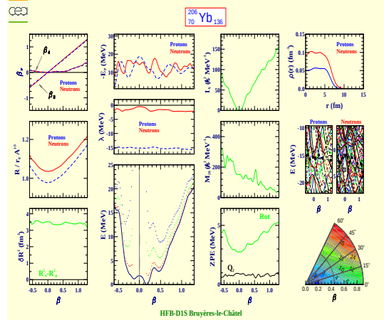
Ytterbium 206 (Z=70, N=136)
