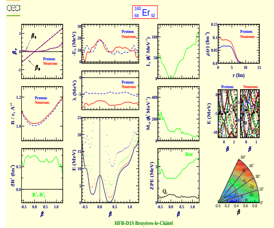
Erbium 160 (Z=68, N=92)
