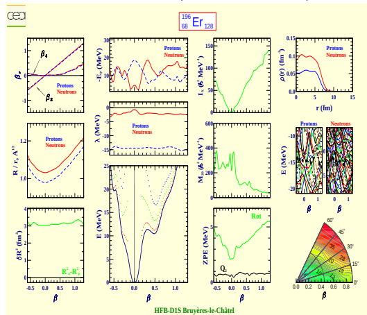
Erbium 196 (Z=68, N=128)
