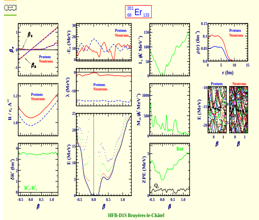
Erbium 201 (Z=68, N=133)
