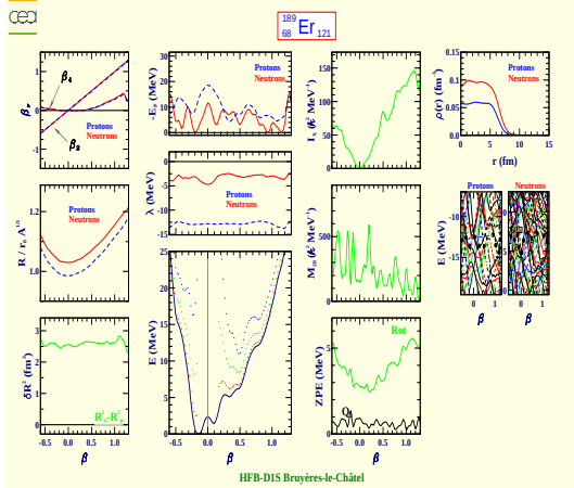
Erbium 189 (Z=68, N=121)
