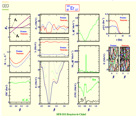
Erbium 195 (Z=68, N=127)
