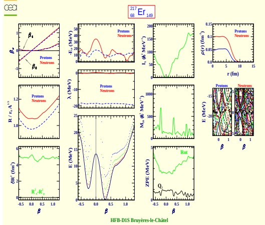
Erbium 217 (Z=68, N=149)
