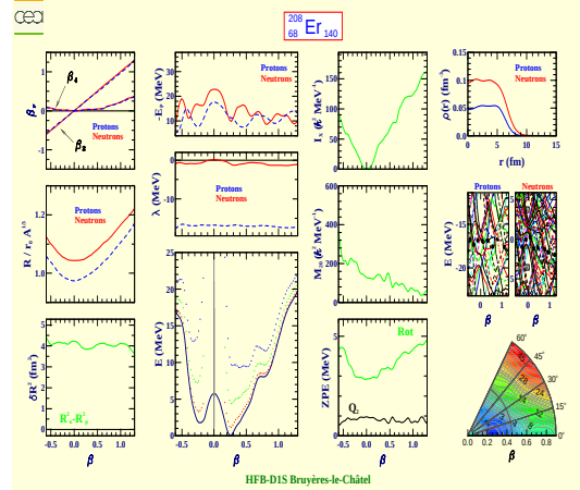
Erbium 208 (Z=68, N=140)
