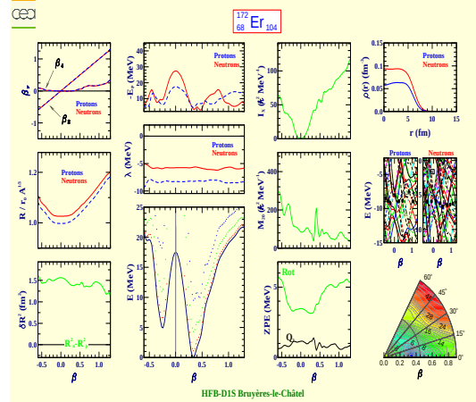
Erbium 172 (Z=68, N=104)
