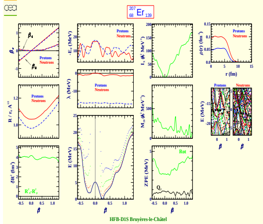
Erbium 207 (Z=68, N=139)
