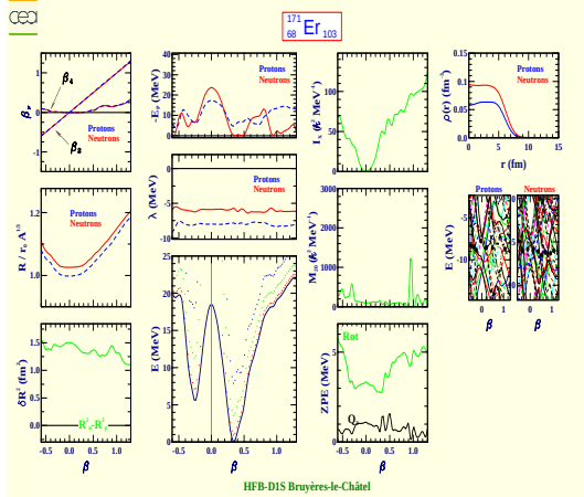
Erbium 171 (Z=68, N=103)
