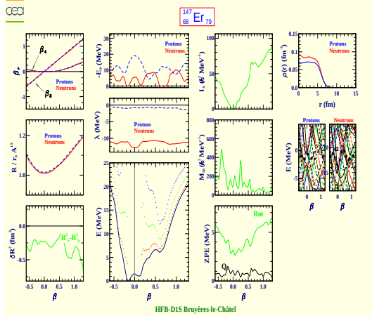
Erbium 147 (Z=68, N=79)
