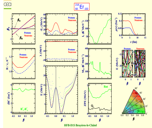
Erbium 218 (Z=68, N=150)
