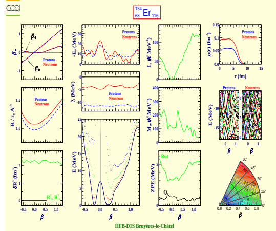
Erbium 184 (Z=68, N=116)
