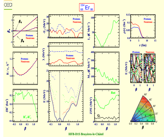
Erbium 154 (Z=68, N=86)
