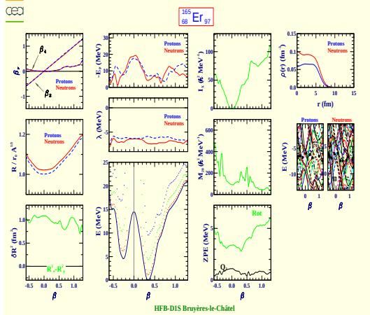
Erbium 165 (Z=68, N=97)
