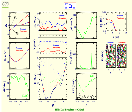
Erbium 153 (Z=68, N=85)
