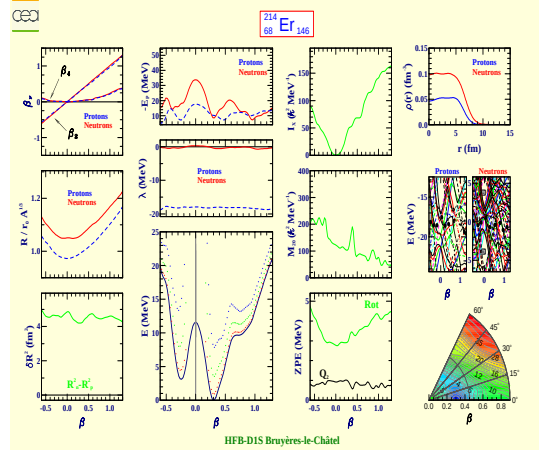
Erbium 214 (Z=68, N=146)
