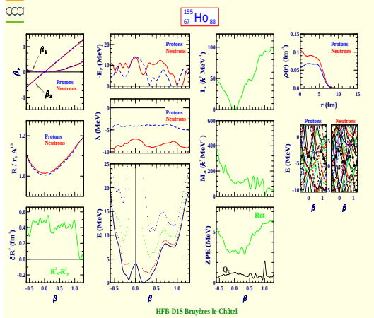
Holmium 155 (Z=67, N=88)
