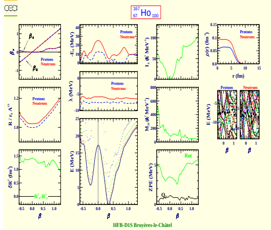
Holmium 167 (Z=67, N=100)
