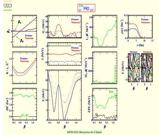
Holmium 174 (Z=67, N=107)
