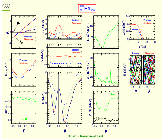
Holmium 173 (Z=67, N=106)
