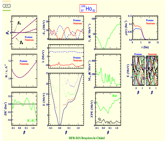
Holmium 149 (Z=67, N=82)
