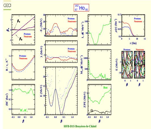
Holmium 162 (Z=67, N=95)
