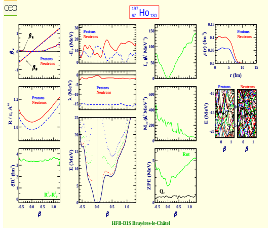
Holmium 197 (Z=67, N=130)
