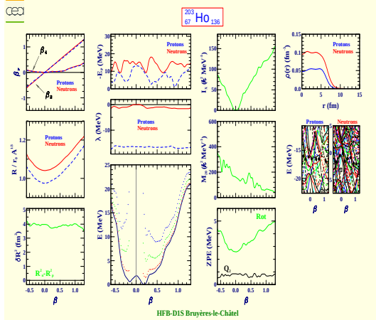
Holmium 203 (Z=67, N=136)
