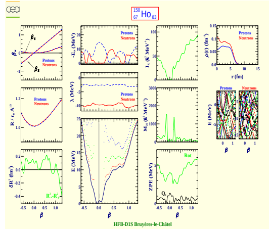
Holmium 150 (Z=67, N=83)
