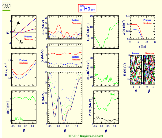
Holmium 179 (Z=67, N=112)
