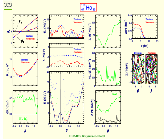
Holmium 156 (Z=67, N=89)
