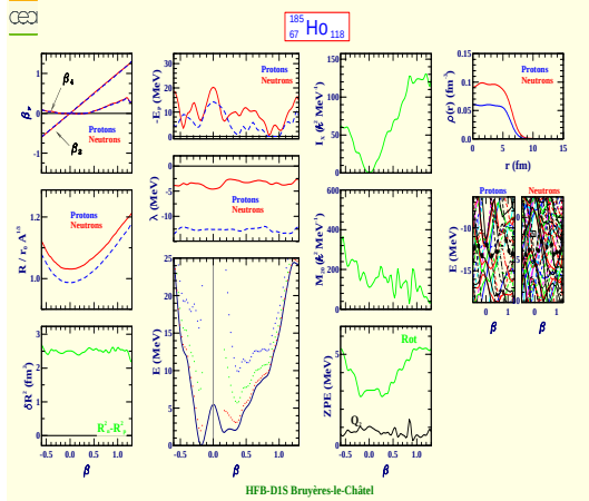
Holmium 185 (Z=67, N=118)
