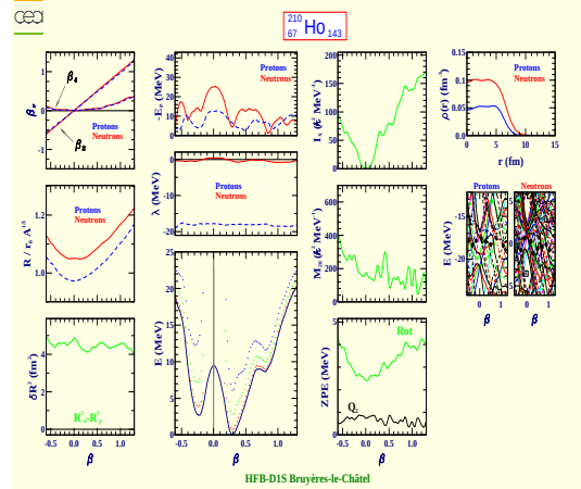
Holmium 210 (Z=67, N=143)
