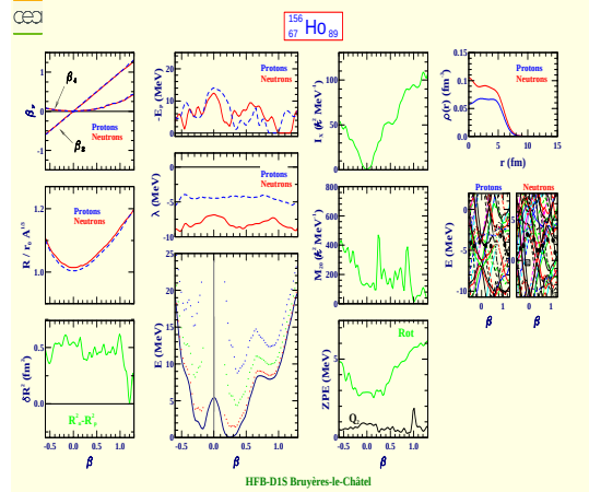
Holmium 156 (Z=67, N=89)
